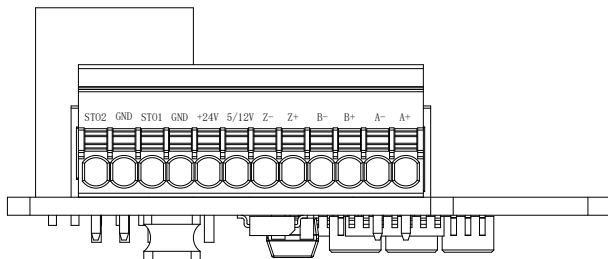
图1-3 端子丝印示意图
