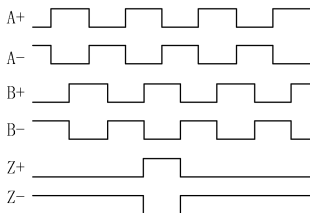
图1-4 ABZ信号
