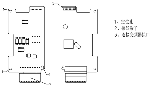
图1-2 PG*1S外观 (5.5kW及以上机型适配)
