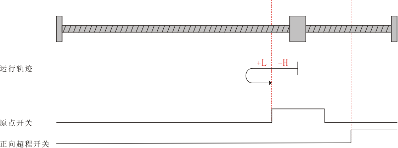
图 6-6 回零模式 0 运行轨迹图 2
