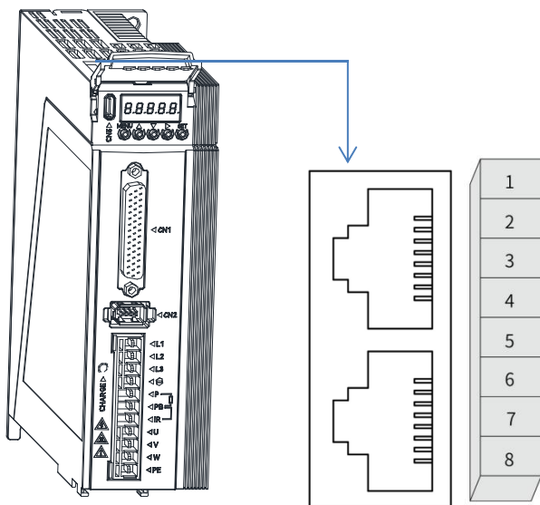
图 4-21 通讯接口连接图
