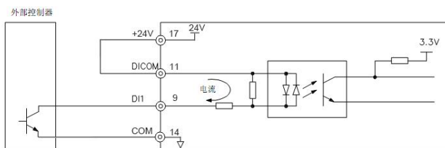
图 4-6 DI 端子 NPN 连接方式（使用伺服驱动器内部 24V 电源）
