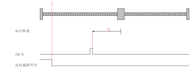
图 6-13 回零模式 3 运行轨迹图 1
