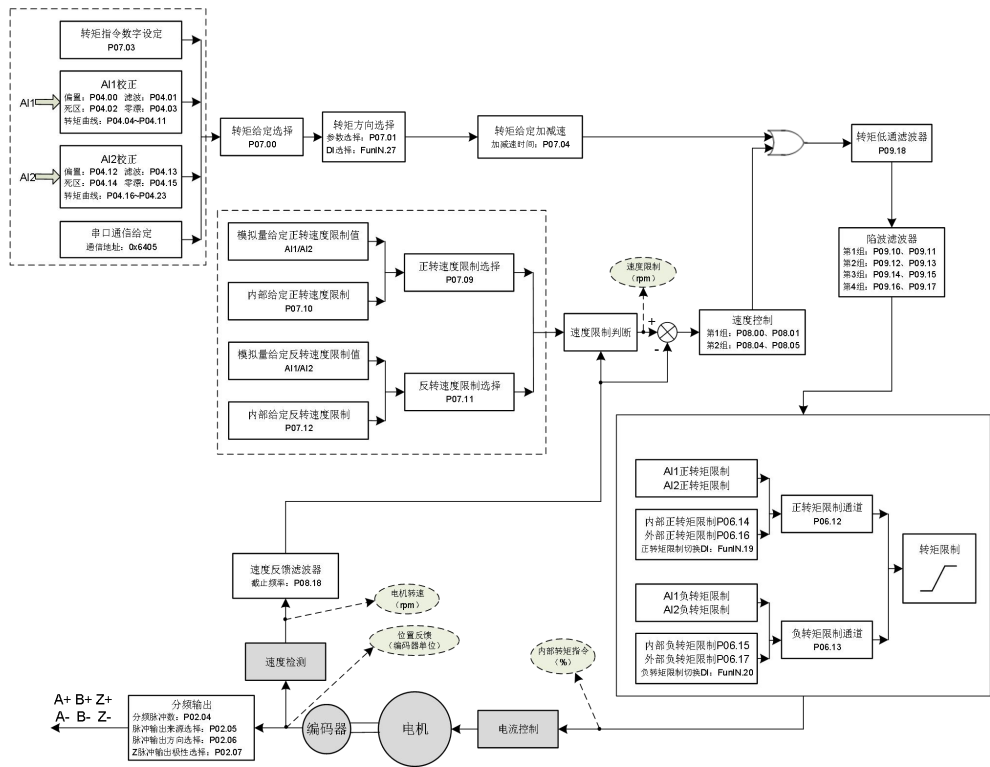
图 6-35 转矩控制模式功能框图
