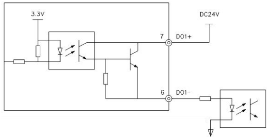
图 4-12 DO 端子源型 (PNP) 输出接线方式
