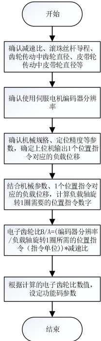
图 6-3 电子齿轮比设置流程
