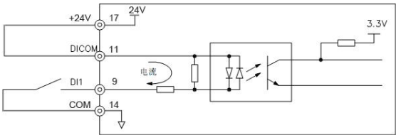
图 4-4 DI 端子干接点连接方式（使用伺服驱动器内部 24V 电源）
