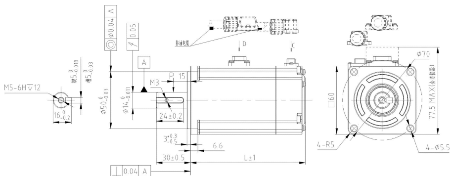
图 2-8 60 框号中惯量伺服电机（ST1-L 系列）外形尺寸图
