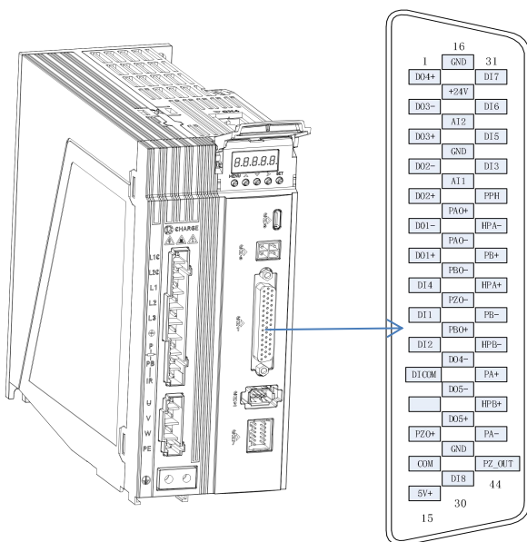
图 4-3 控制信号端子定义图 (SIZE D)
