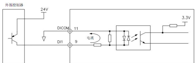
图 4-9 DI 端子 PNP 连接方式（使用外部电源）
