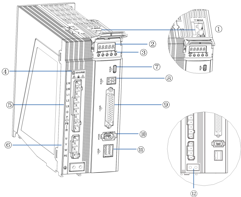
图 1-7 M5-P 伺服驱动器各部分示意图 (M5-PS012A、M5-PS016A、M5-PT3R5A、M5-PT5R4A、M5-PT8R4A、M5-PT012A)
