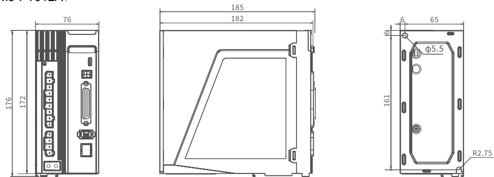
图 2-3 SIZE D 伺服驱动器外形尺寸图
