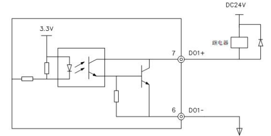
图 4-10 DO 端子连接继电器接线方式
