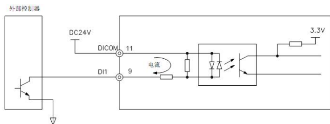
图 4-7 DI 端子 NPN 连接方式（使用外部电源）
