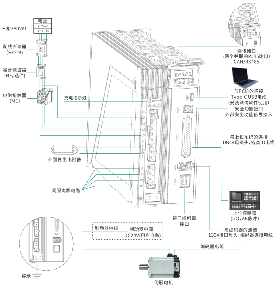
图 3-7 SIZE D 三相 380V 伺服系统配线图
