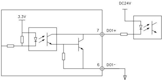
图 4-11 DO 端子漏型 (NPN) 输出接线方式
