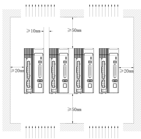
保留间距安装
