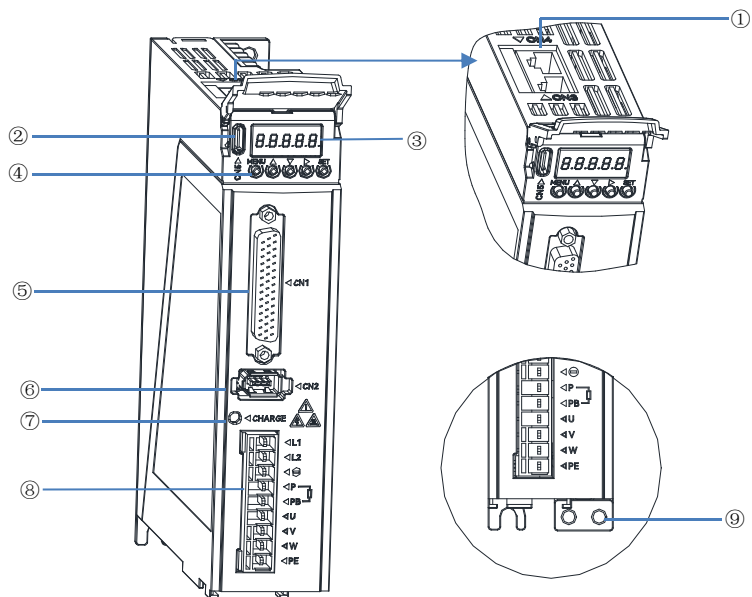
图 1-5 M5-P 伺服驱动器各部分示意图（M5-PS1R6A、M5-PS2R8A）
