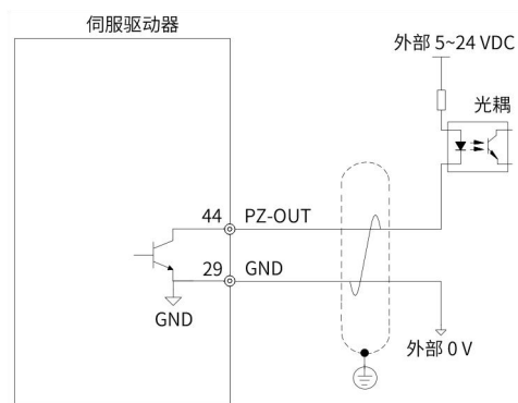
图 4-20 编码器分频输出接线图 3
