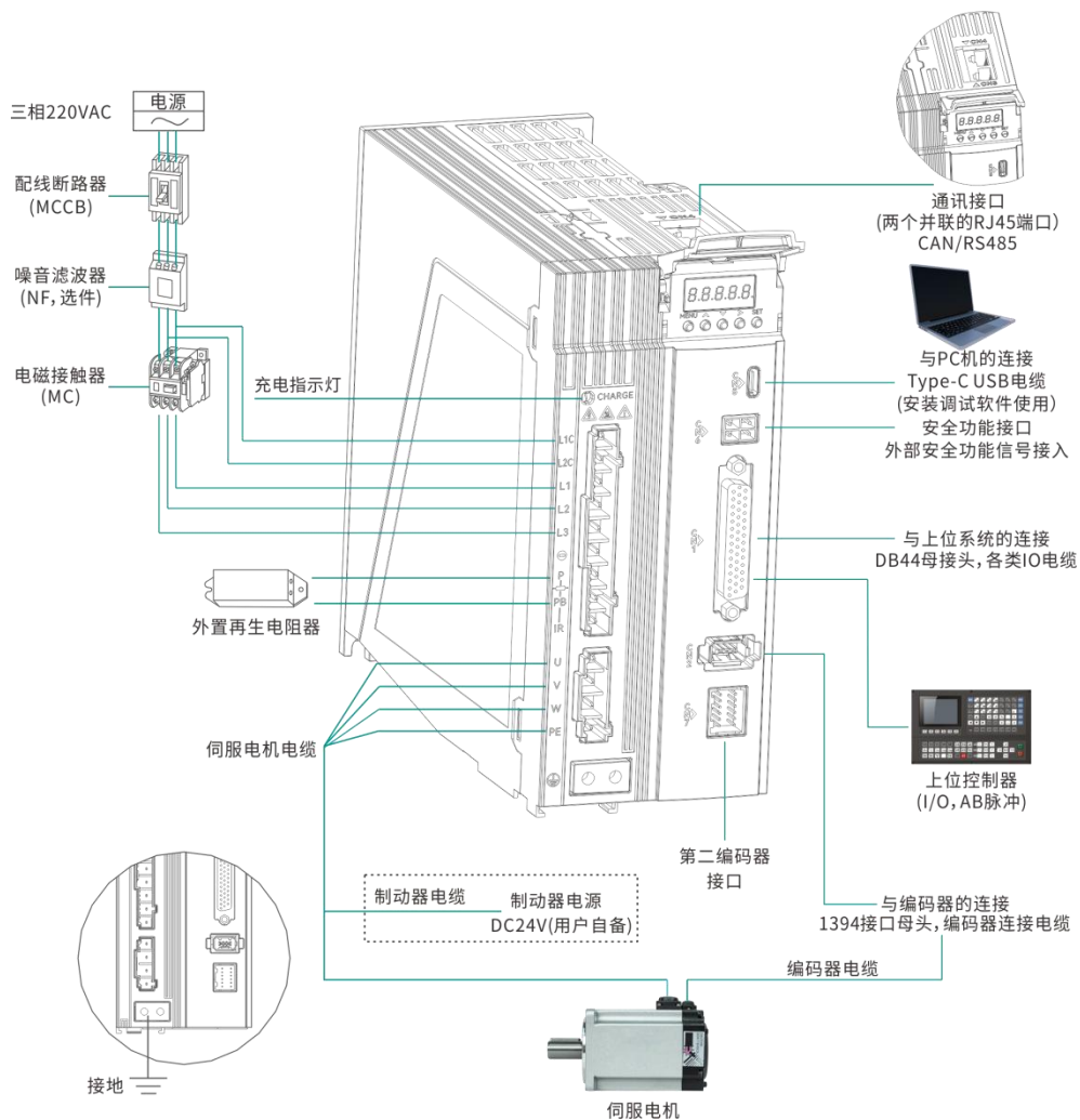
图 3-6 SIZE D 三相 220V 伺服系统配线图
