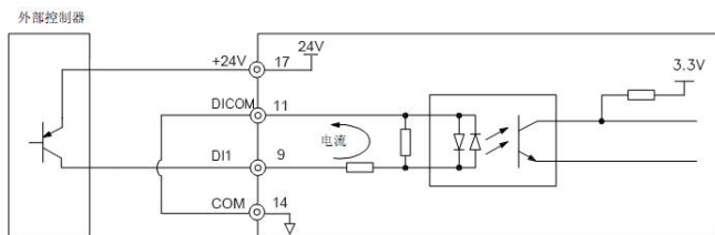
图 4-8 DI 端子 PNP 连接方式（使用伺服驱动器内部 24V 电源）
