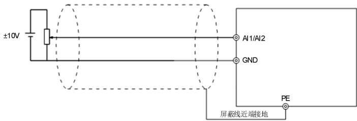
图 4-13 AI1/AI2 单端电压输入配线图
