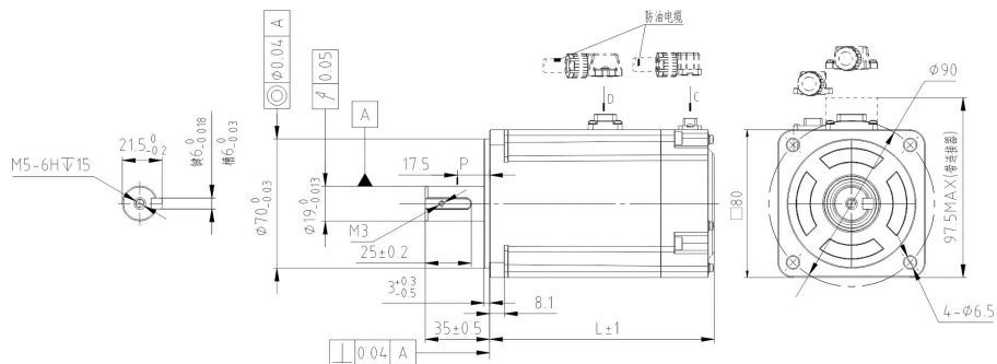
图 2-9 80 框号中惯量伺服电机（ST1-L 系列）外形尺寸图
