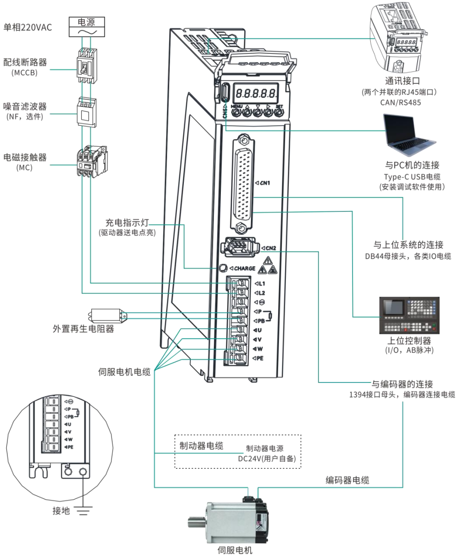
图 3-4 SIZE A 单相 220V 伺服系统配线图
