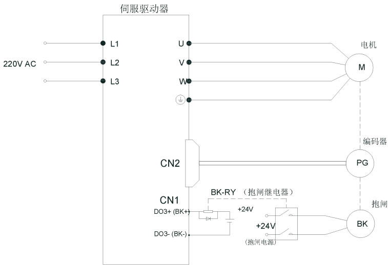
图 6-36 抱闸配线图
