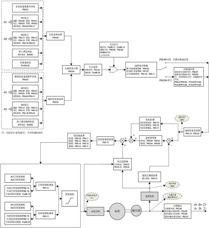
图 6-33 速度控制模式功能框图
