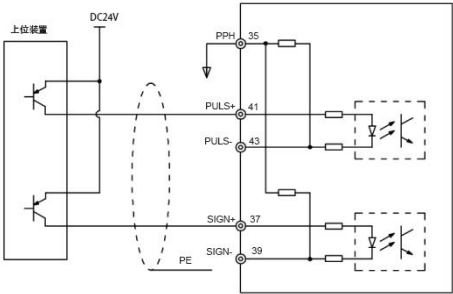
图 4-16 低速脉冲指令 PNP 输入接线图
