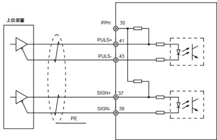
图 4-14 低速脉冲指令差分输入接线图
