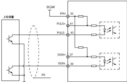
图 4-15 低速脉冲指令 NPN 输入接线图
