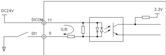
图 4-5 DI 端子干接点连接方式（使用外部电源）
