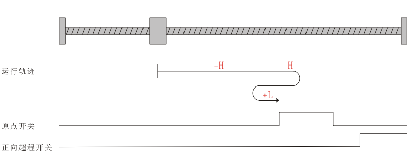
图 6-5 回零模式 0 运行轨迹图 1
