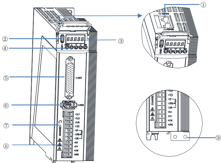
图 1-6 M5-P 伺服驱动器各部分示意图（M5-PS5R5A、M5-PS7R6A）
