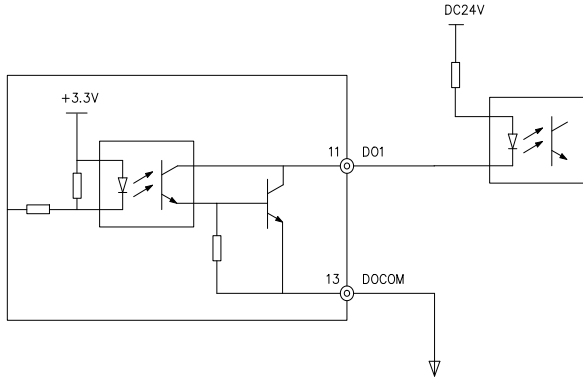
图 4-7 DO 端子漏型（NPN）输出接线方式
