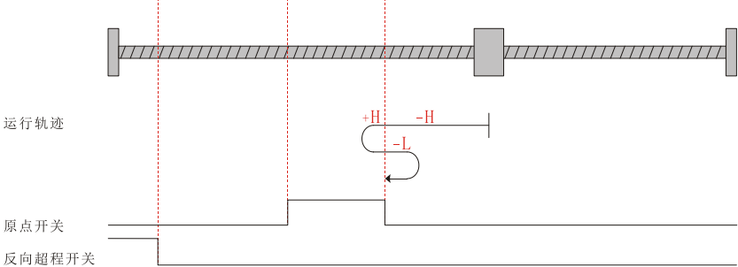
图 5-10 回零模式 1 运行轨迹图 3
