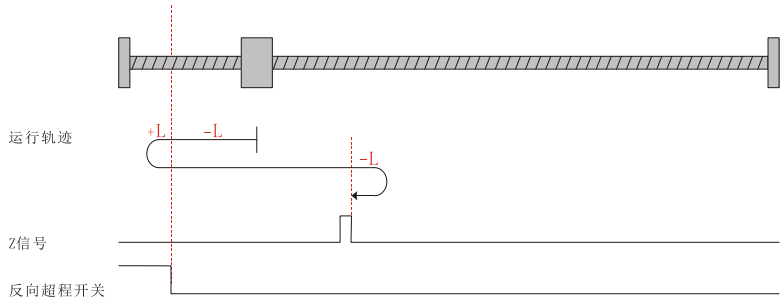
图 5-14 回零模式 3 运行轨迹图 2
