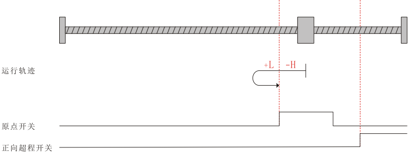
图 5-6 回零模式 0 运行轨迹图 2
