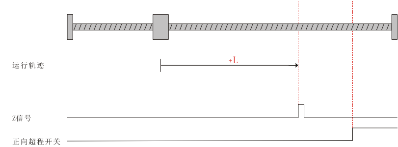
图 5-11 回零模式 2 运行轨迹图 1
