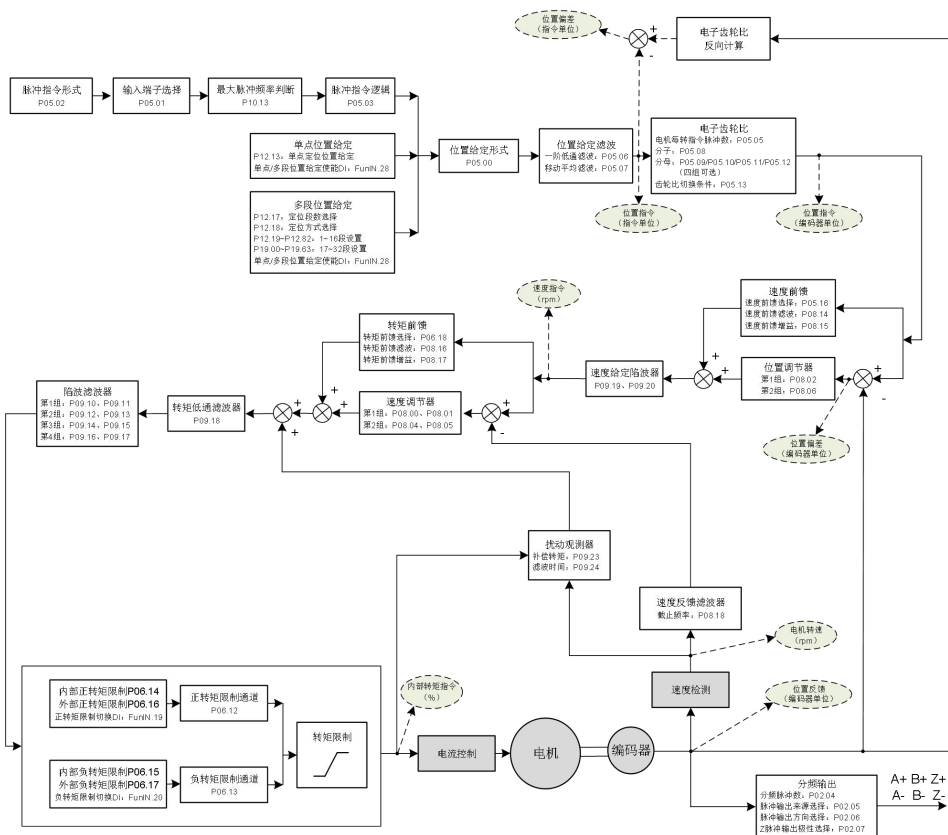
图 5-30 位置控制模式功能框图
