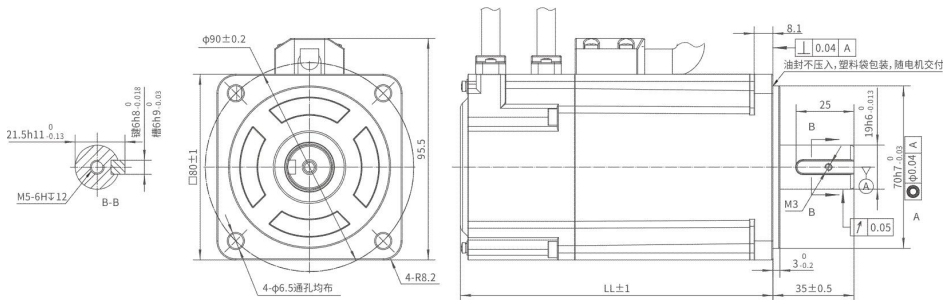
图 2-7 80 框号伺服电机外形尺寸图二 (带抱闸)
