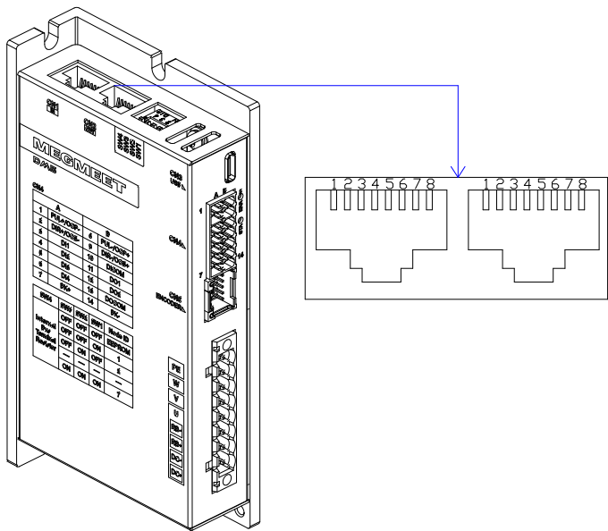
图 4-12 通讯接口连接图
