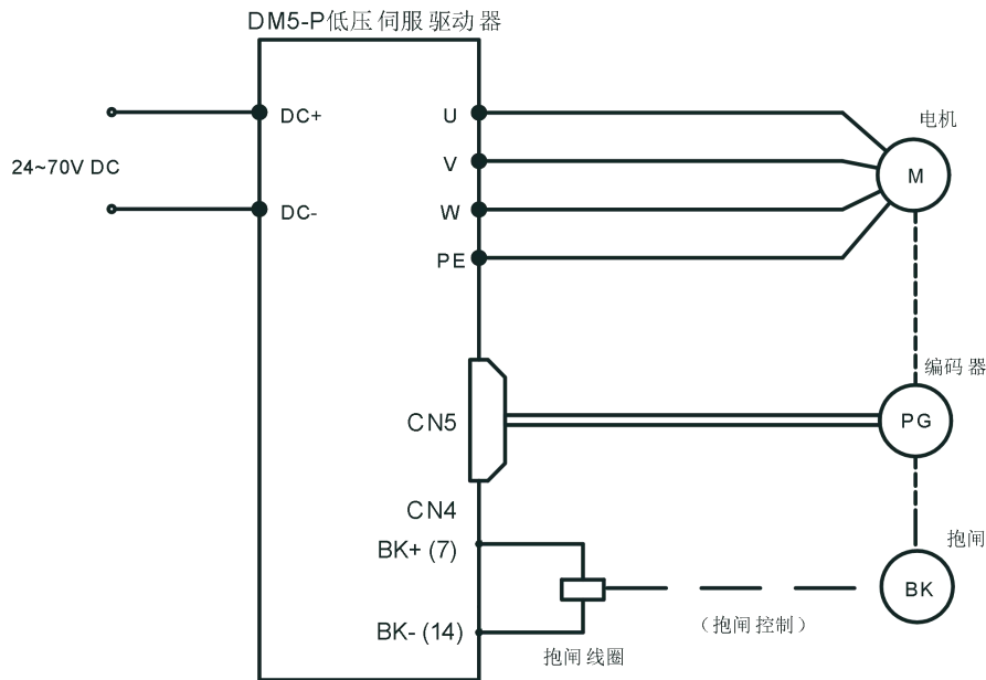
图 5-36 抱闸配线图
