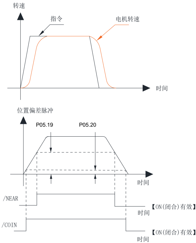
图 5-2 定位接近和定位完成信号逻辑
