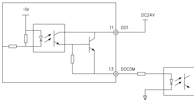
图 4-8 DO 端子源型 (PNP) 输出接线方式
