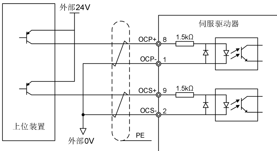
图 4-11 脉冲指令 PNP 输入接线图
