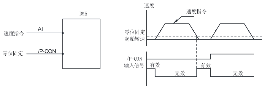
图 5-32 零位固定逻辑
