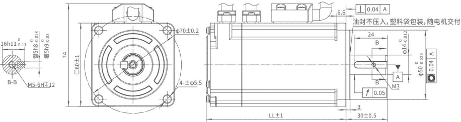
图 2-5 60 框号伺服电机外形尺寸图（带抱闸）
