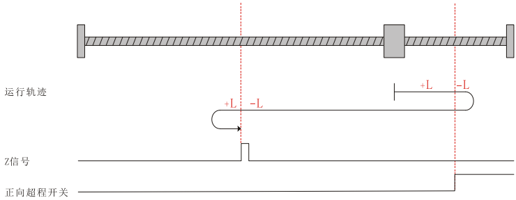
图 5-12 回零模式 2 运行轨迹图 2
