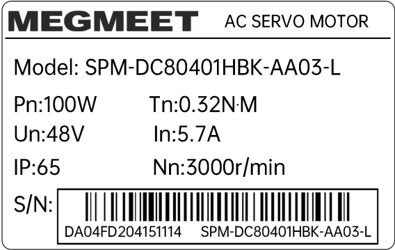
图 1-2 DM5 伺服电机铭牌说明
