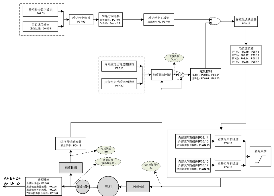
图 5-35 转矩控制模式功能框图
