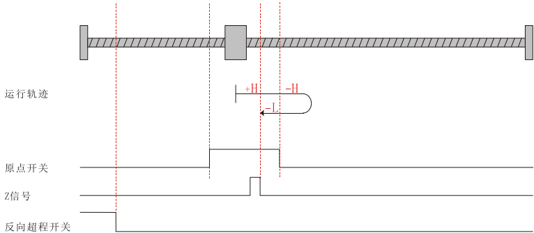
图 5-19 回零模式 5 运行轨迹图 2
