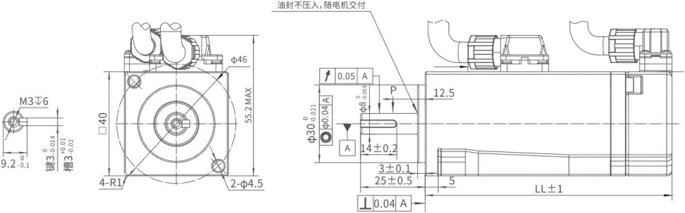
图 2-3 40 框号伺服电机外形尺寸图
