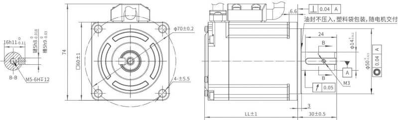
图 2-4 60 框号伺服电机外形尺寸图（不带抱闸）
