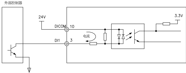
图 4-4 DI 端子 NPN 连接方式
