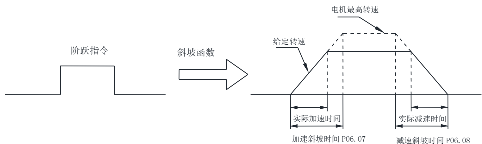
图 5-31 指令斜坡函数工作逻辑
