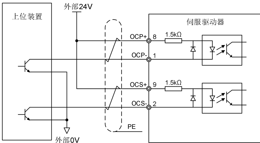
图 4-10 脉冲指令 NPN 输入接线图
