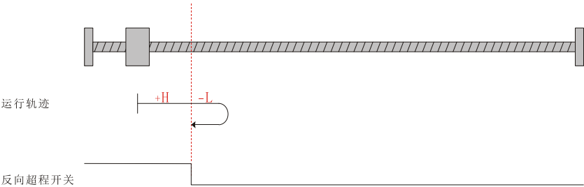
图 5-24 回零模式 7 运行轨迹图 2
