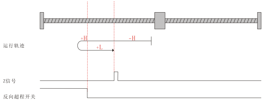
图 5-27 回零模式 9 运行轨迹图 1
