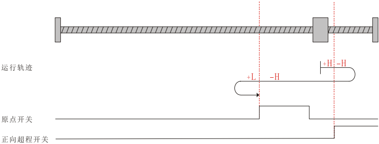
图 5-7 回零模式 0 运行轨迹图 3
