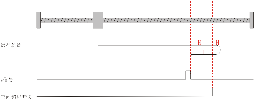
图 5-25 回零模式 8 运行轨迹图 1
