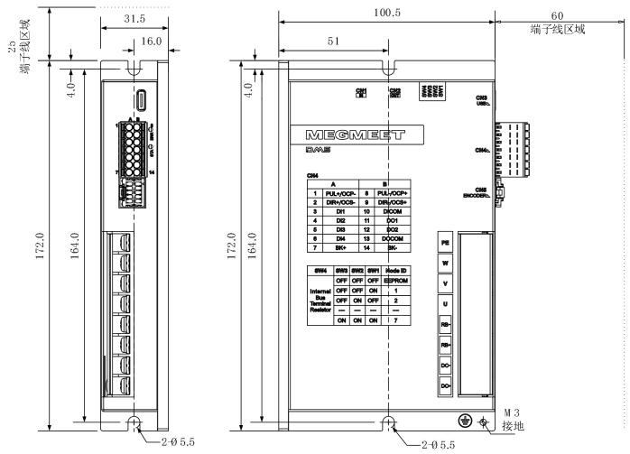
图 2-2 SIZE B 伺服驱动器外形尺寸图
