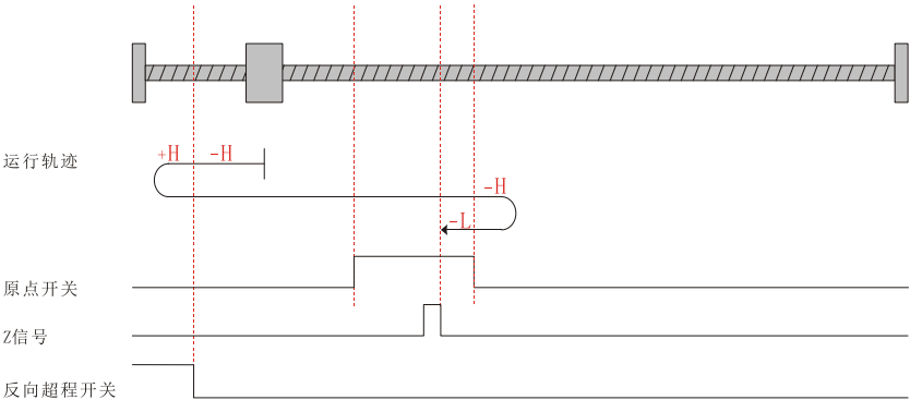
图 5-18 回零模式 5 运行轨迹图 1
