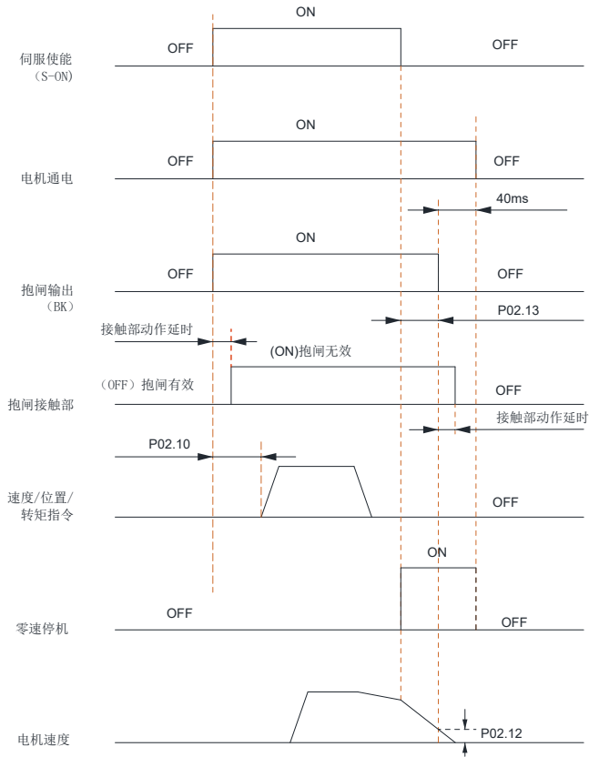
图 5-38 电机旋转时抱闸时序图
