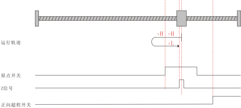
图 5-16 回零模式 4 运行轨迹图 2
