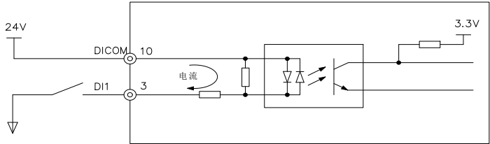
图 4-3 DI 端子干接点连接方式
