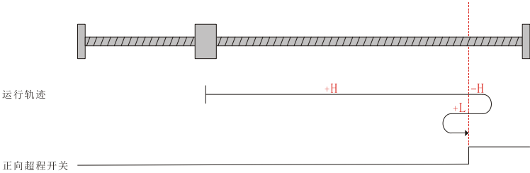
图 5-21 回零模式 6 运行轨迹图 1
