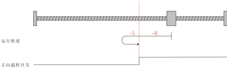
图 5-22 回零模式 6 运行轨迹图 2
