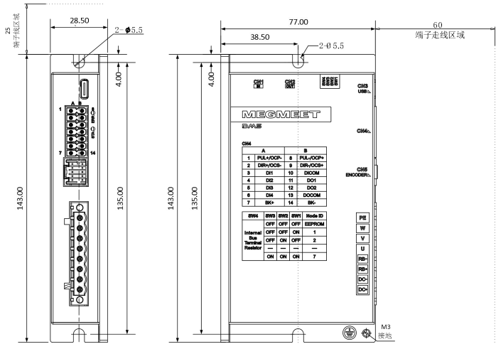
图 2-1 SIZE A 伺服驱动器外形尺寸图
