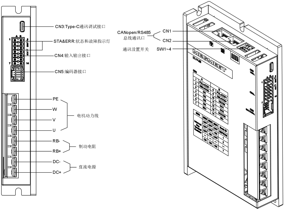
图 1-6 DM5-P 伺服驱动器各部分示意图（SIZE B）
