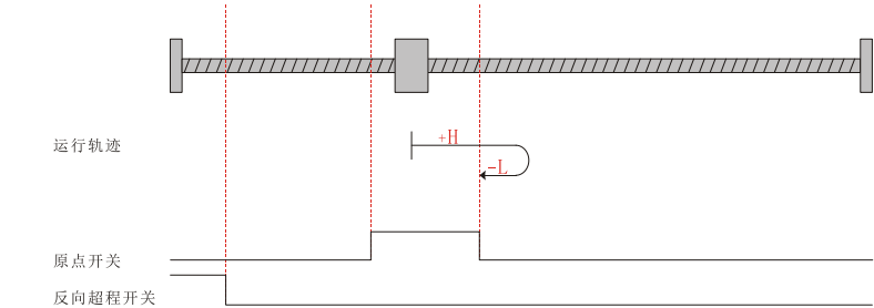
图 5-9 回零模式 1 运行轨迹图 2
