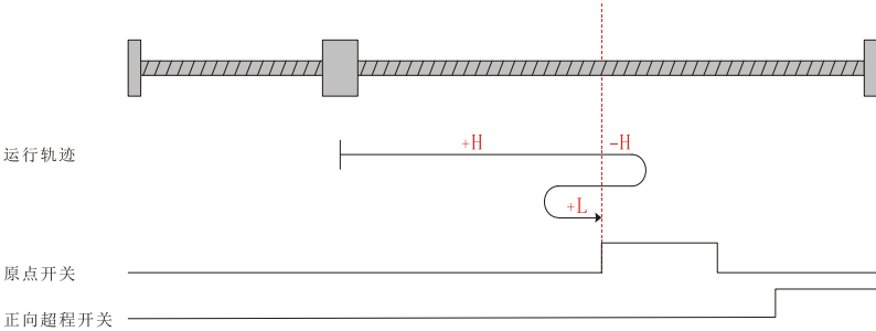
图 5-5 回零模式 0 运行轨迹图 1
