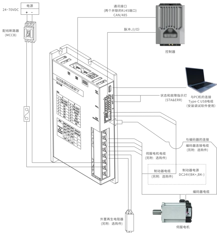
图 3-3 SIZE B 伺服系统配线图
