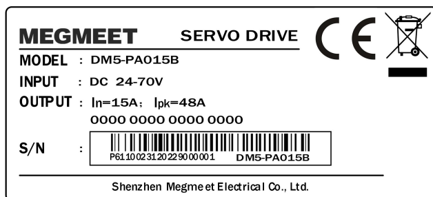
图 1-4 DM5-P 伺服驱动器铭牌说明
