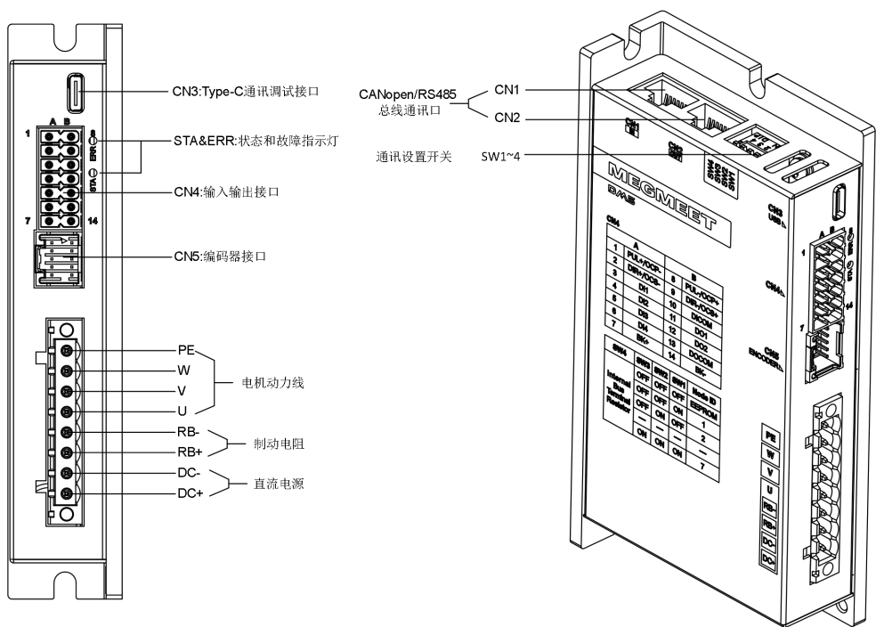
图 1-5 DM5-P 伺服驱动器各部分示意图 (SIZE A)
