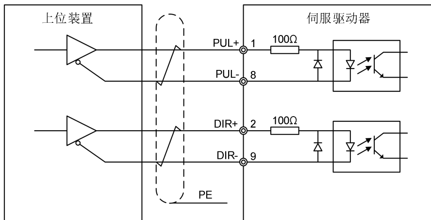
图 4-9 脉冲指令差分输入接线图
