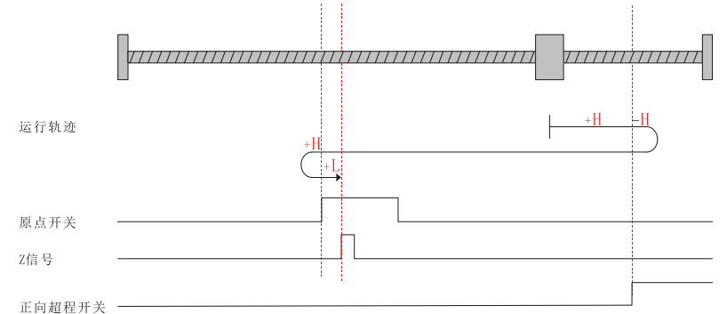
图 5-17 回零模式 4 运行轨迹图 3
