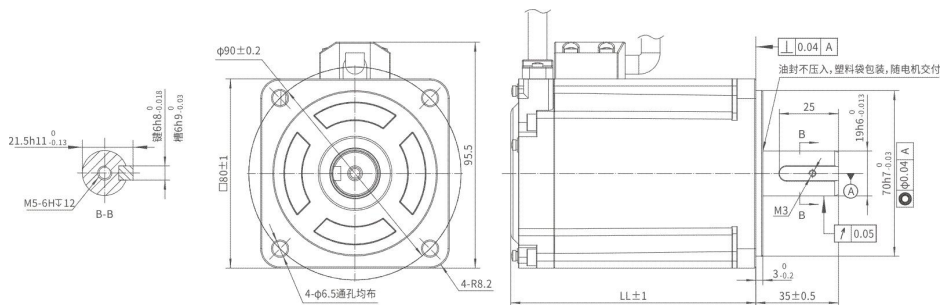
图 2-6 80 框号伺服电机外形尺寸图一（不带抱闸）
