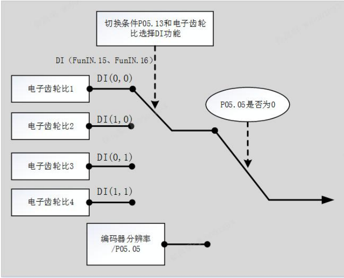
图 5-4 电子齿轮比功能示意图
