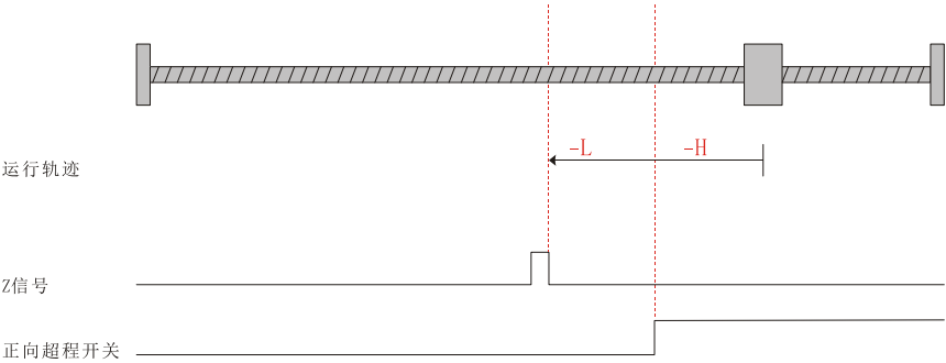
图 5-26 回零模式 8 运行轨迹图 2
