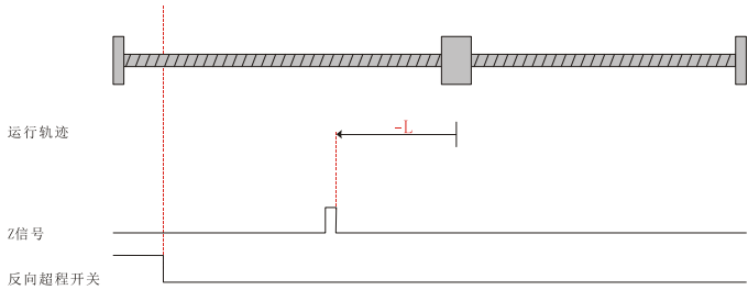
图 5-13 回零模式 3 运行轨迹图 1
