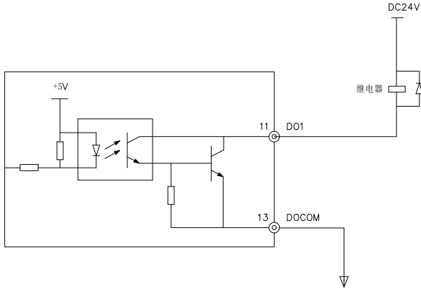
图 4-6 DO 端子连接继电器接线方式
