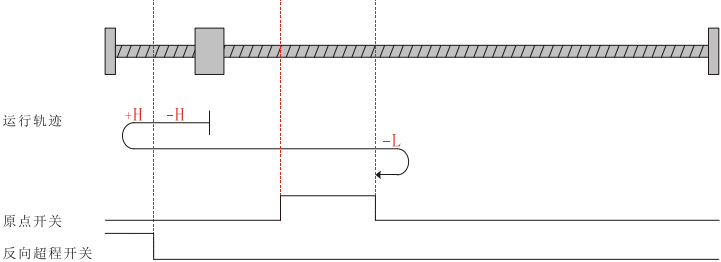
图 5-8 回零模式 1 运行轨迹图 1
