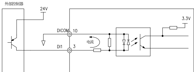
图 4-5 DI 端子 PNP 连接方式
