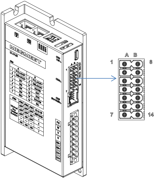
图 4-2 控制信号端子定义图
