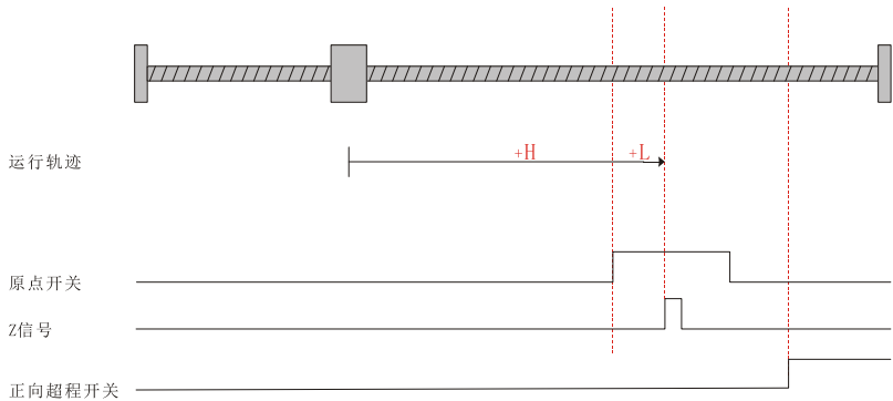
图 5-15 回零模式 4 运行轨迹图 1
