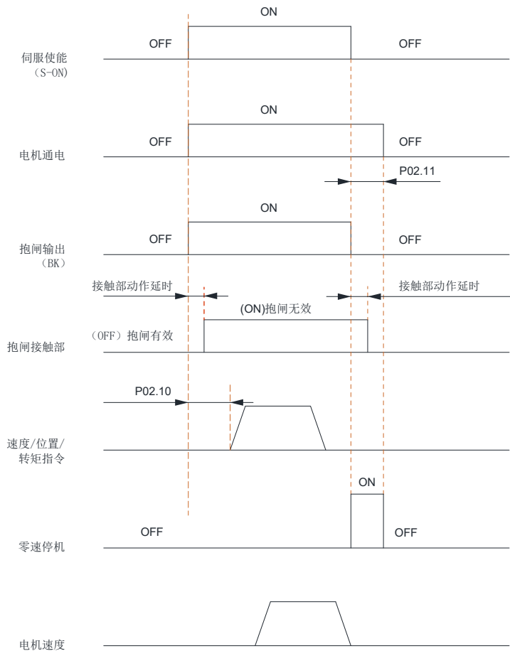
图 5-37 电机静止时抱闸时序图
