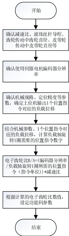
图 5-3 电子齿轮比设置流程
