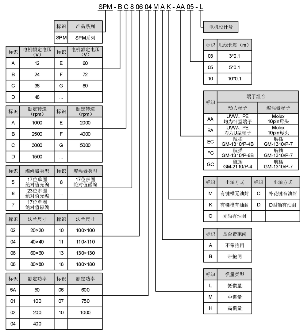
图 1-1 DM5 伺服电机型号说明
