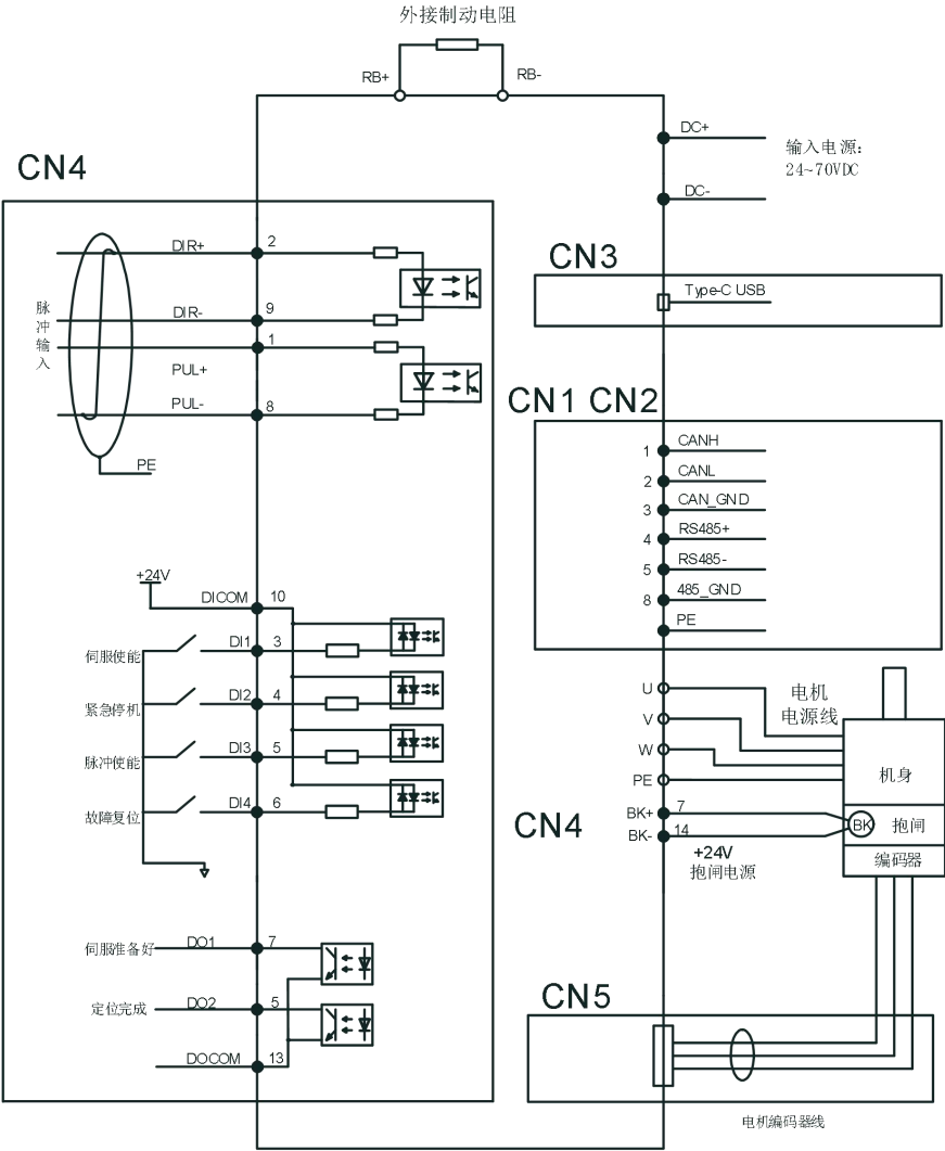
图 5-1 位置控制模式接线图
