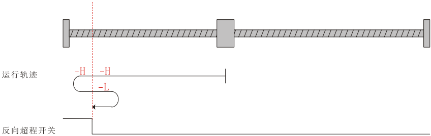
图 5-23 回零模式 7 运行轨迹图 1
