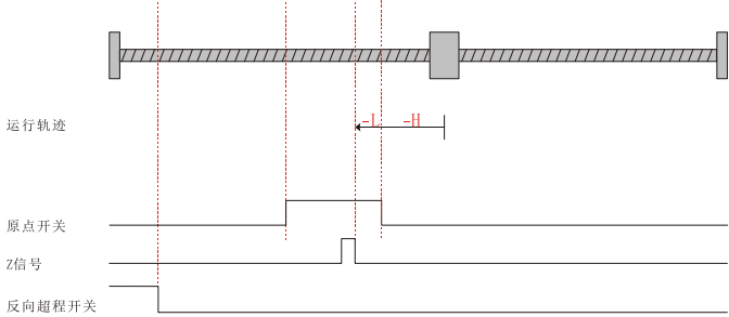
图 5-20 回零模式 5 运行轨迹图 3
