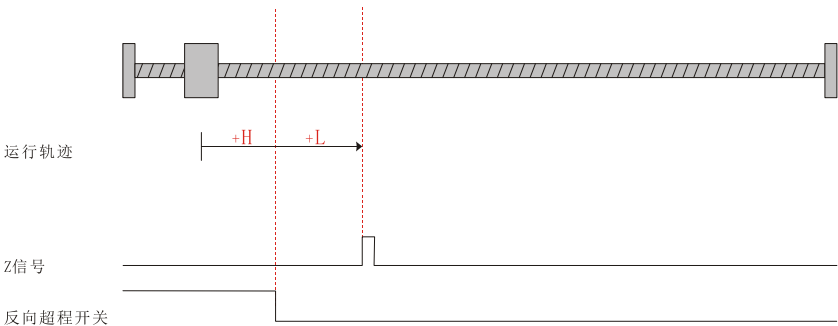
图 5-28 回零模式 9 运行轨迹图 2
