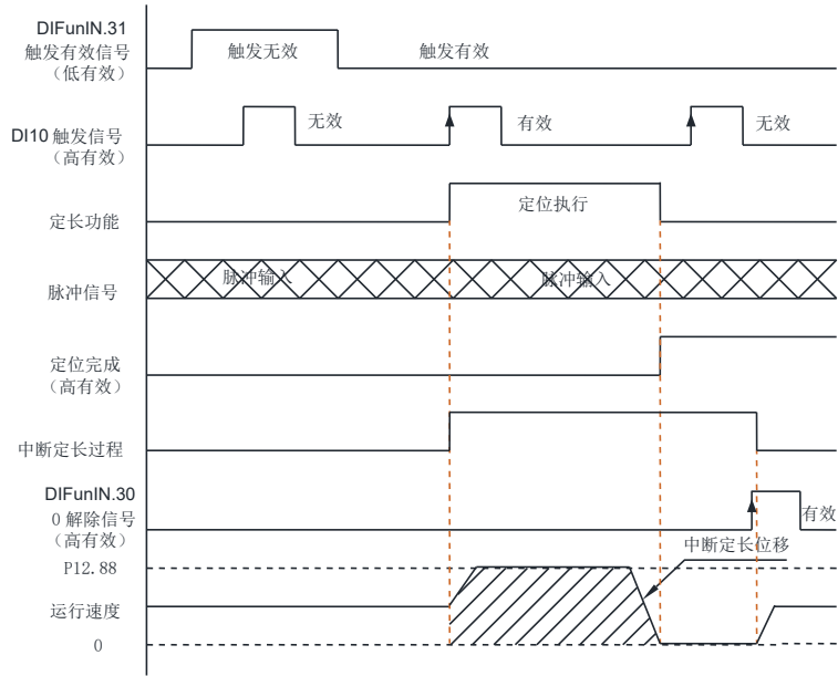
图 5-29 中断定长时序图
