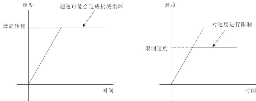
图 5-34 转矩控制速度限幅
