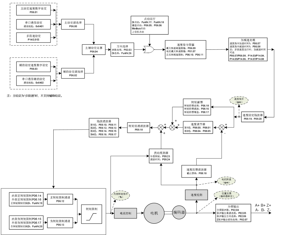
图 5-33 速度控制模式功能框图
