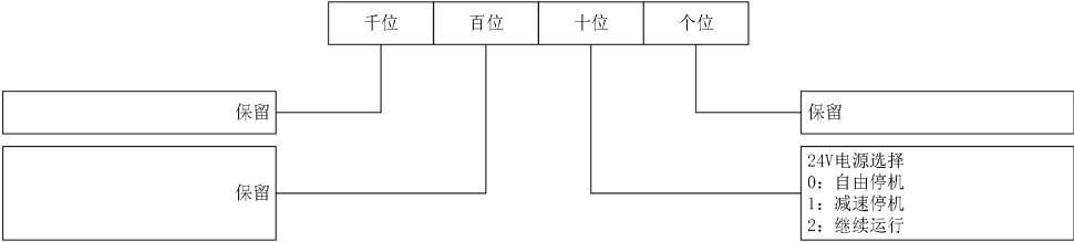
图7-55 故障保护属性设定4
