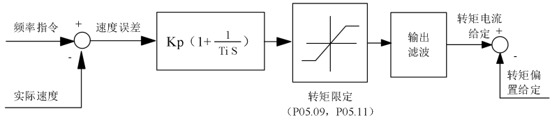
图7-10 速度调节器简化图
