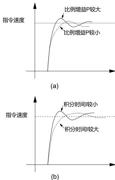
图7-11 阶跃响应与PI关系图
