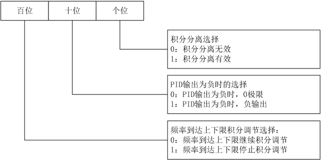
图7-46 PID输出特性选择
