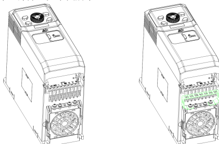
图2-41 绑线架
