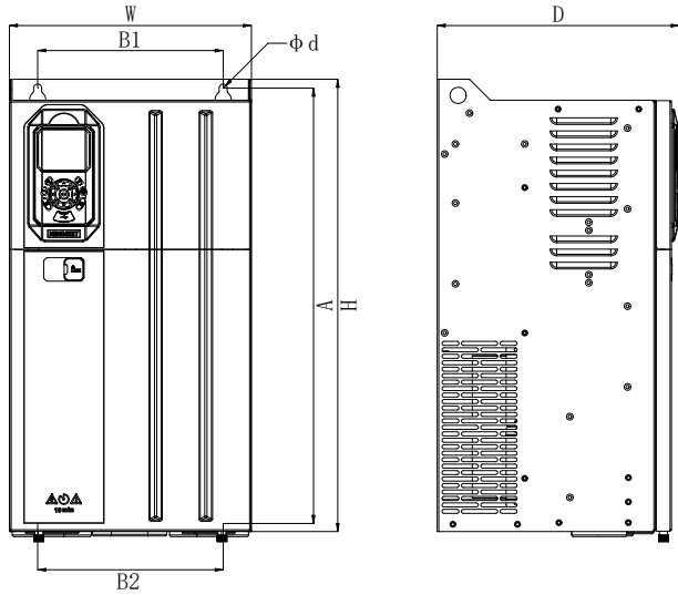
图 1-8 箱体 H
