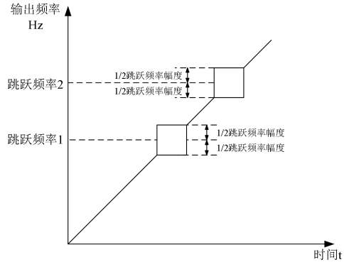
图7-31
