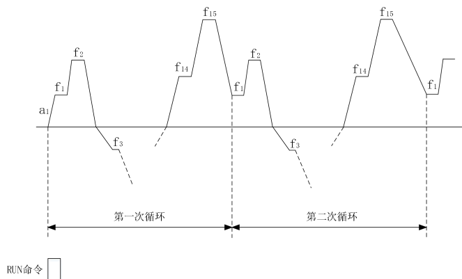
图7-38 PLC连续循环方式
