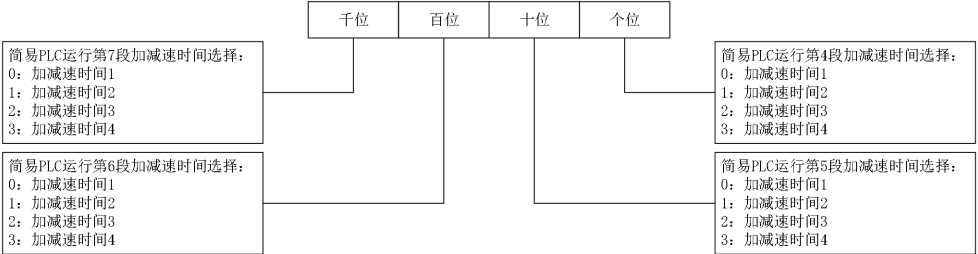
图7-41 简易PLC第4～7段加减速时间选择
