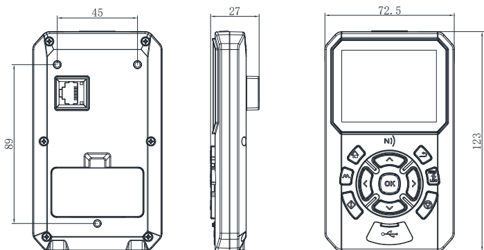
图2-51 大型远程LCD键盘/操作面板（单位：mm）
