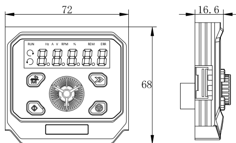
图2-47 远程LED键盘/操作面板
