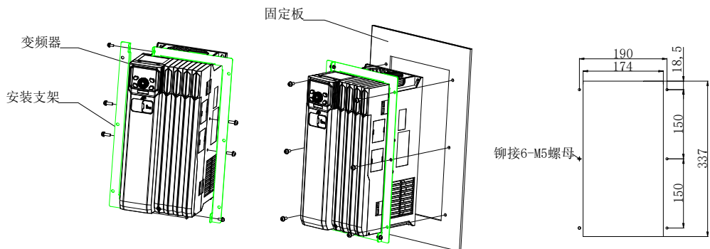
图2-36 MV810-EMBE (适用于18.5~22kW)
