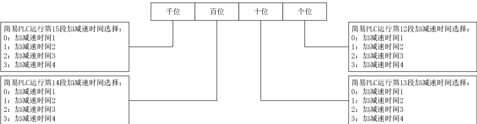
图7-43 简易PLC第12～15段加减速时间选择
