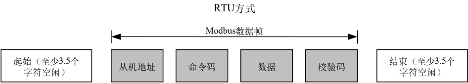
图附 1-1 Modbus 协议格式
