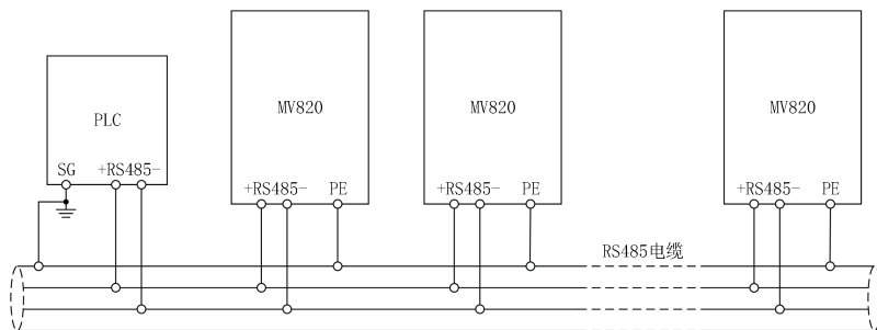
图 4-14 PLC 与变频器多机通讯时推荐的接线图（变频器、电机全部良好接地）
