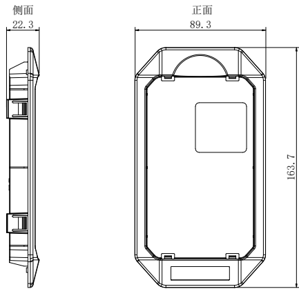
图2-45 大型键盘安装底座（单位：mm）
