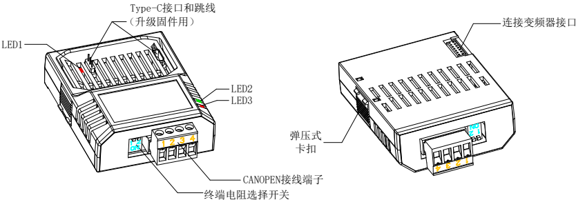
图2-13 端子部件示意图
