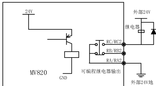
图 4-21 继电器输出端子接线方式
