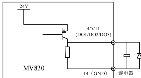
图 4-20 多功能输出端子 D0 接线方式
