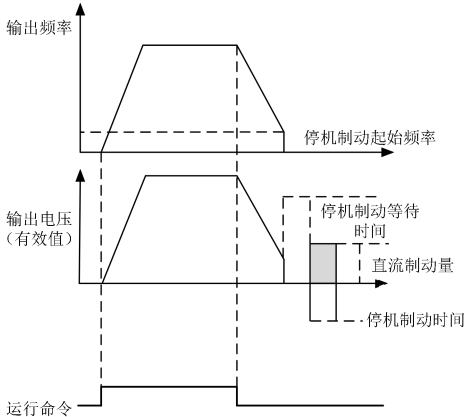
图7-17 减速停车+直流制动示意图
