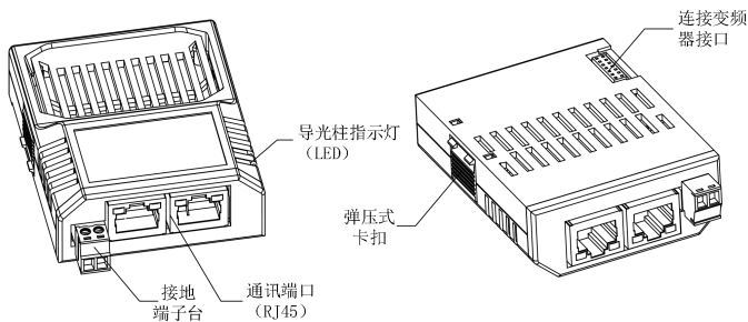
图2-7 端子部件示意图
