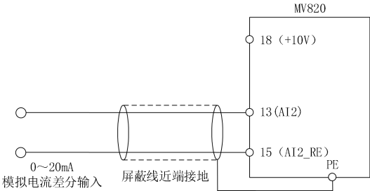
图 4-8 13 端子电流差分输入配线图
