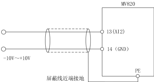
图 4-9 13 端子电压单端输入配线图
