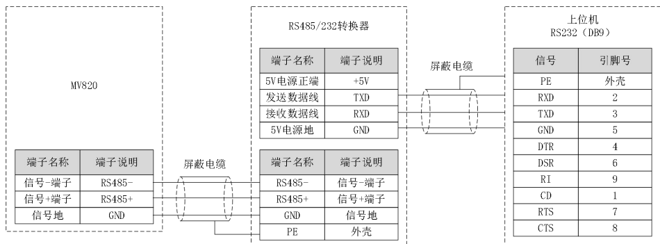
图 4-13 485- (RS485/232) -RS232 通讯配线
