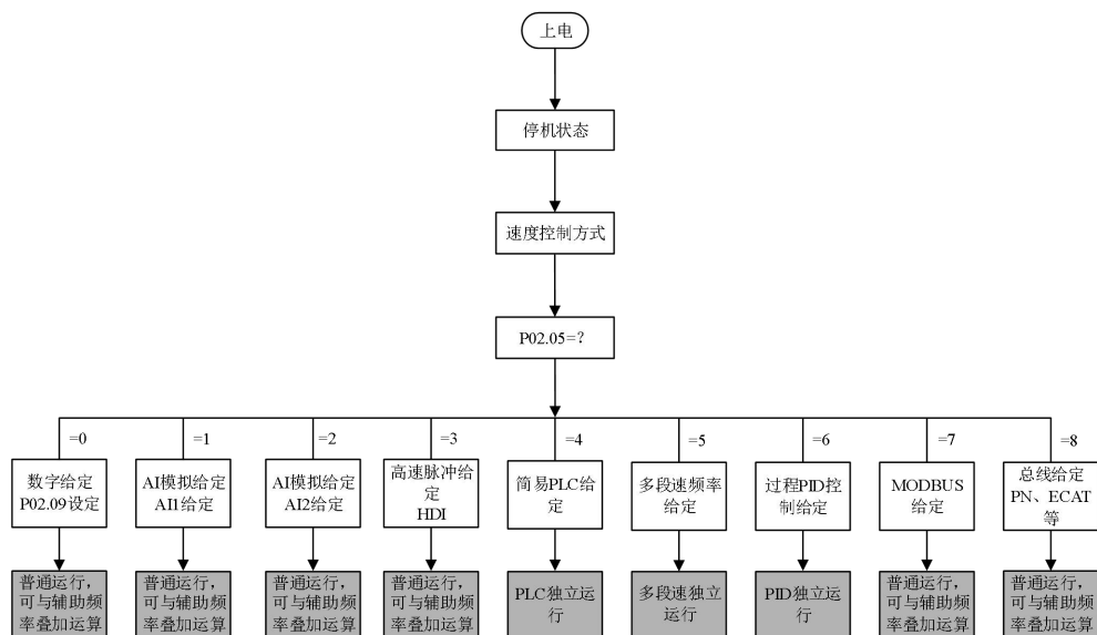
图 5-9 速度控制模式下运行方式选择
