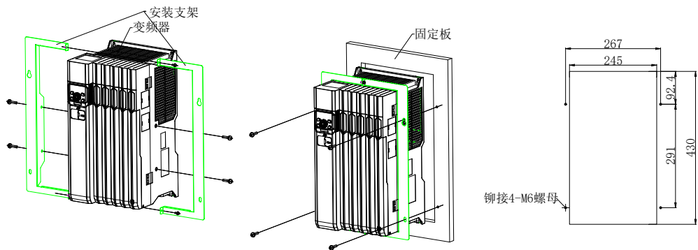
图2-37 MV810-EMBF (适用于30、37kW)
