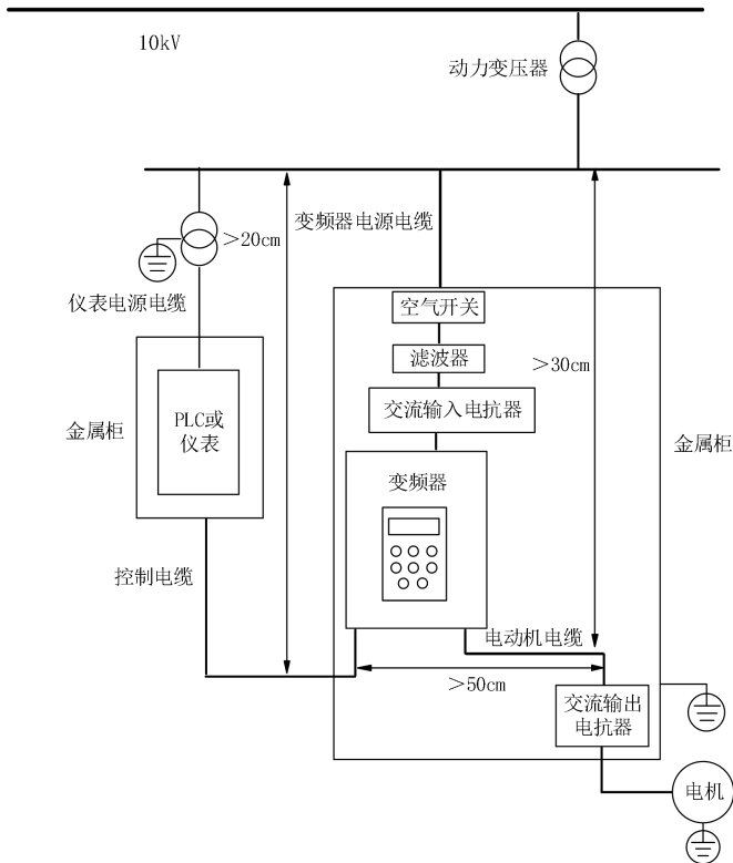
图 4-39 变频器的安装示意图
