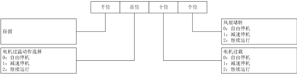
图7-54 故障保护属性设定3
