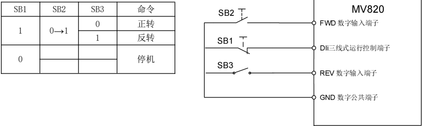
图7-22 三线式运转模式2
