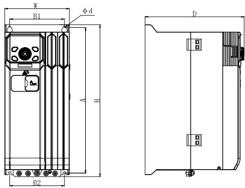
图 1-3 箱体 C
