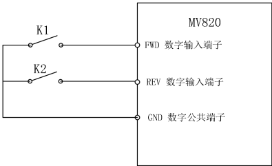
图7-20 两线式控制模式2
