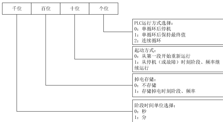
图7-35 简易PLC运行方式选择
