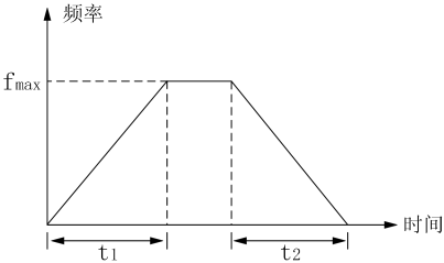
图7-26 直线加减速
