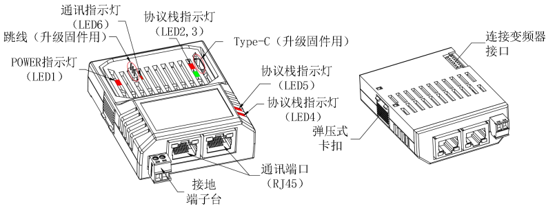
图2-8 端子部件示意图
