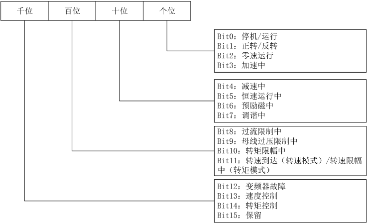
图7-2 变频器运行状态
