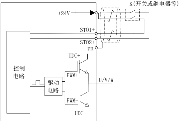
图附3-2 ST0功能电路接线
