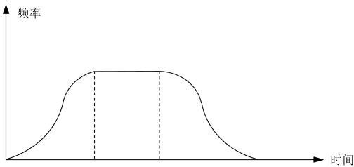
图7-27 S曲线加减速
