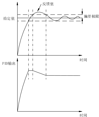
图7-45 偏差极限示意图
