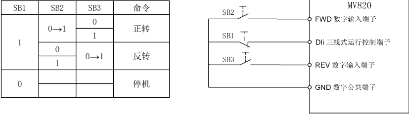
图7-21 三线式运转模式1
