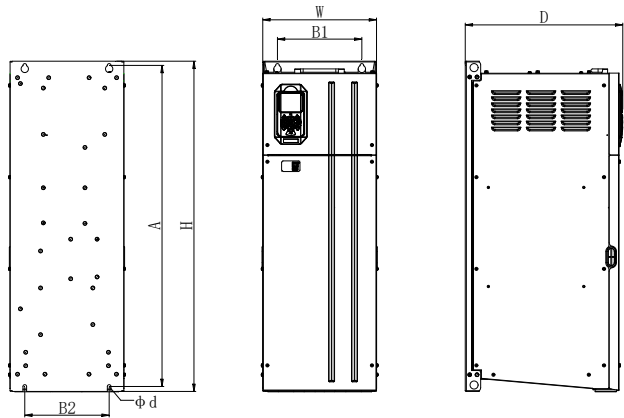
图 1-9 箱体 I
