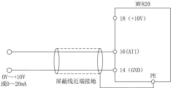
图 4-7 16 端子单端输入配线图
