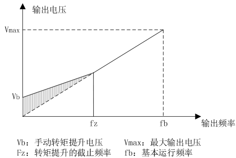
图7-16 转矩提升（提升量为阴影部分）
