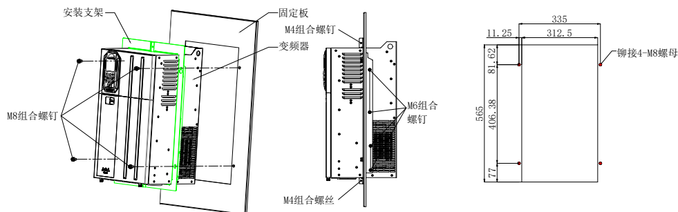
图2-39 MV810-EMBH（适用于90~110kW）
