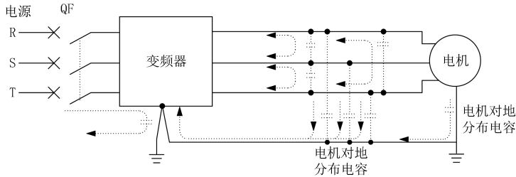
图 4-36 漏电流路径
