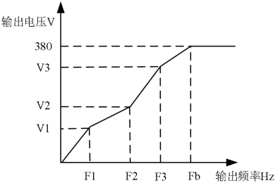
图 7-15 多点 V/F 曲线
