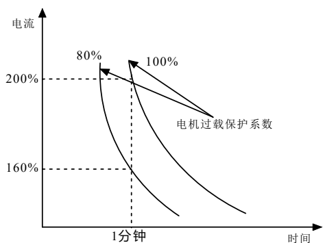
图7-8 电机过载保护系数设定
