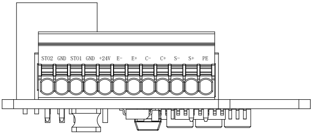
图2-30 端子丝印示意图
