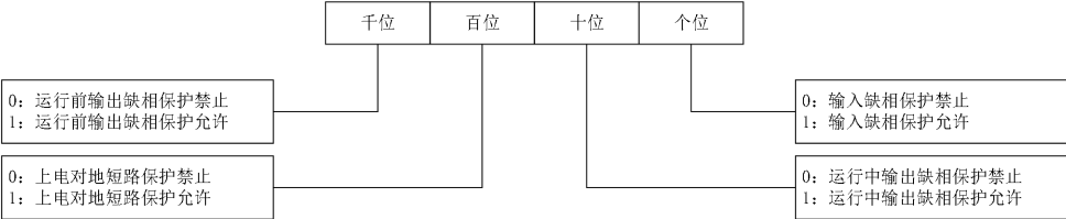
图7-51 输入、输出缺相保护设定
