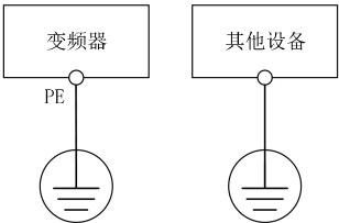
图 4-31 接地示意图 1
