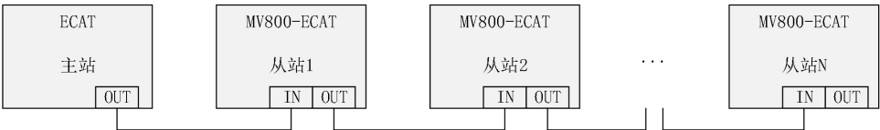
图2-10 ECAT总线连接示意图
