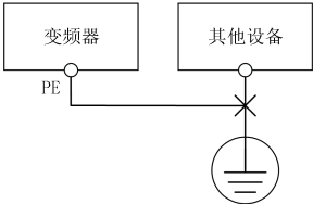
图 4-33 接地示意图 3
