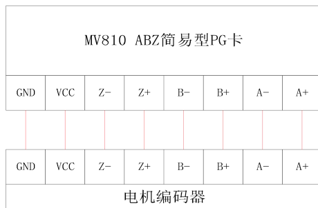
图 10-2 差分接法
