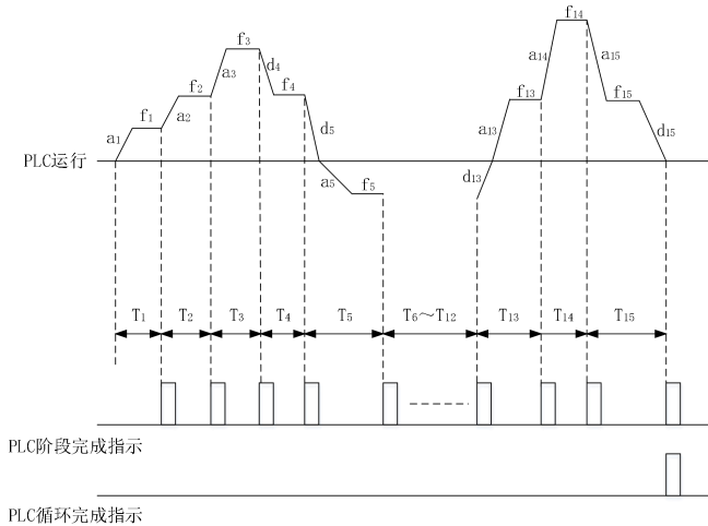
图7-34 简易PLC运行图
