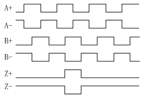
图2-24 ABZ信号
