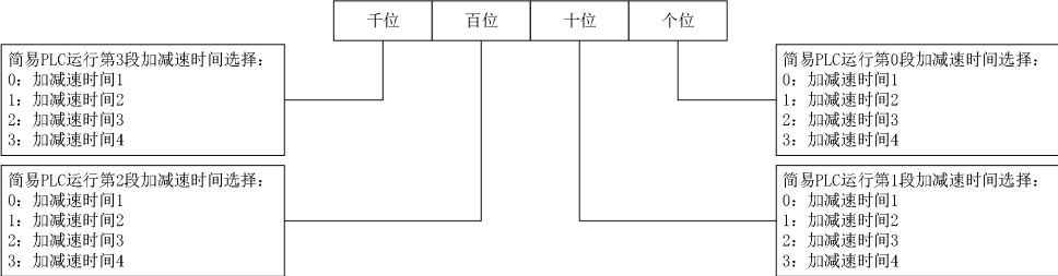
图7-40 简易PLC第0~3段加减速时间选择
