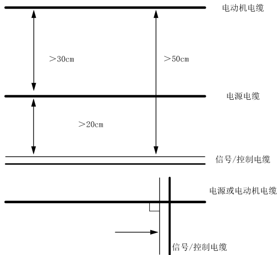
图 4-28 系统配线要求
