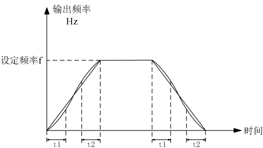
图7-28 S曲线开始、结束段时间比例
