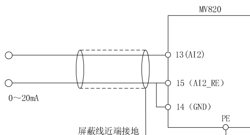
图 4-10 13 端子电流单端输入配线图
