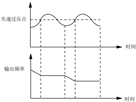
图7-50 过压失速功能
