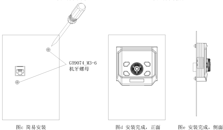
图2-48 远程LED键盘/操作面板简易安装方法
