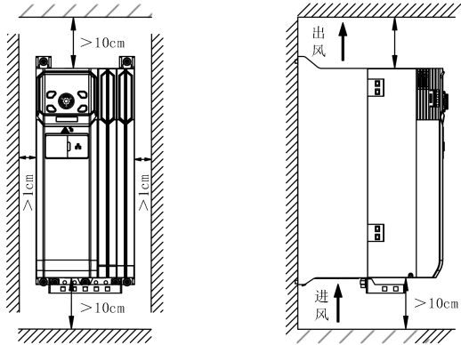
图 3-2 立式安装间隔距离
