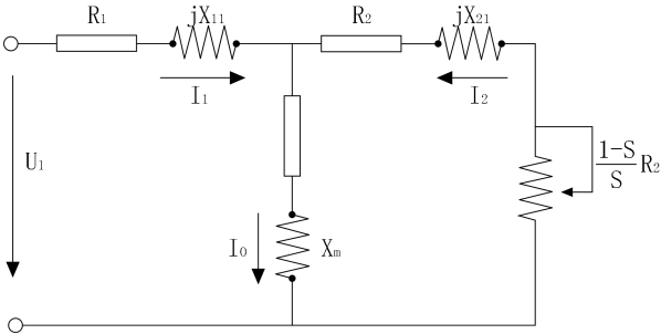
图7-7 异步电机稳态等效电路图
