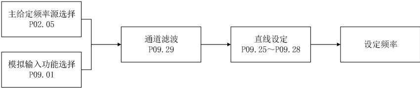
图7-24 给定通道输入与设定频率的关系
