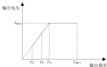
图7-6 极限频率参数定义示意图
