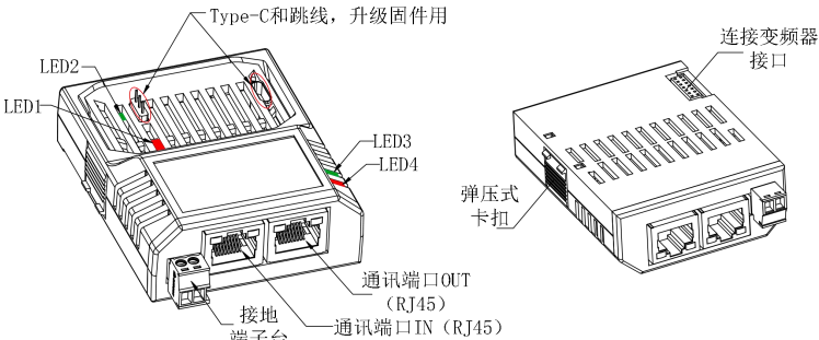
图2-11 端子部件示意图
