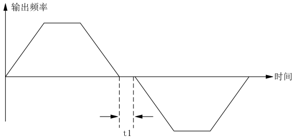
图7-18 正反转死区时间
