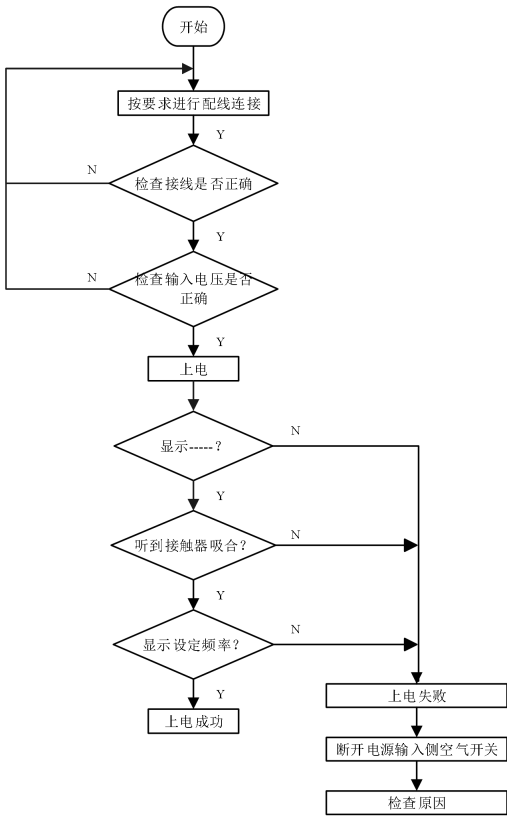
图 5-10 变频器首次上电操作流程
