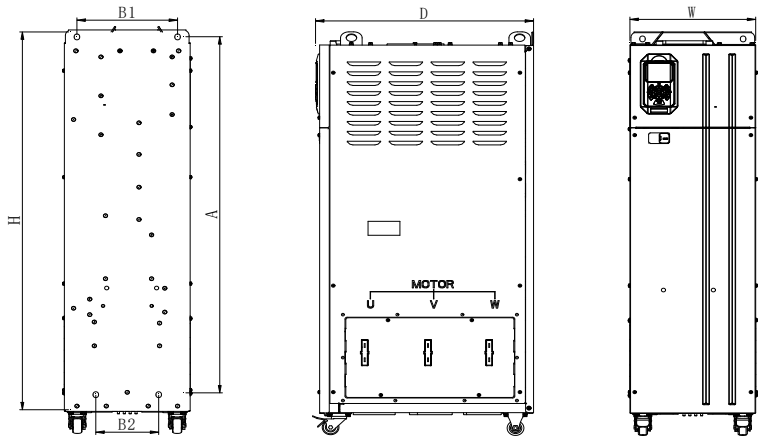
图 1-10 箱体 J
