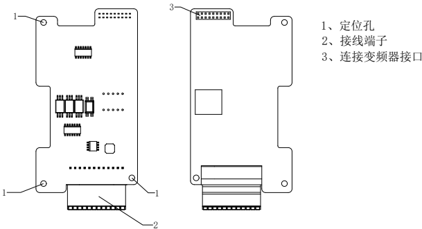
图2-28 PG*2S外观 (3.7kW及以下机型适配)
