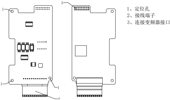
图2-29 PG*2S外观 (5.5kW及以上机型适配)
