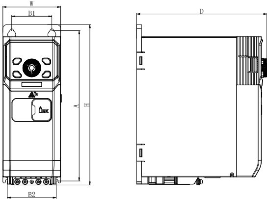
图 1-2 箱体 B
