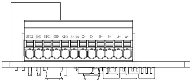
图2-23 端子丝印示意图
