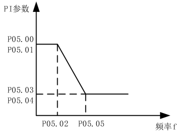
图7-9 PI参数示意图
