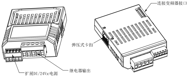
图2-17 端子部件示意图
