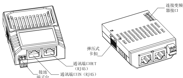
图2-9 端子部件示意图
