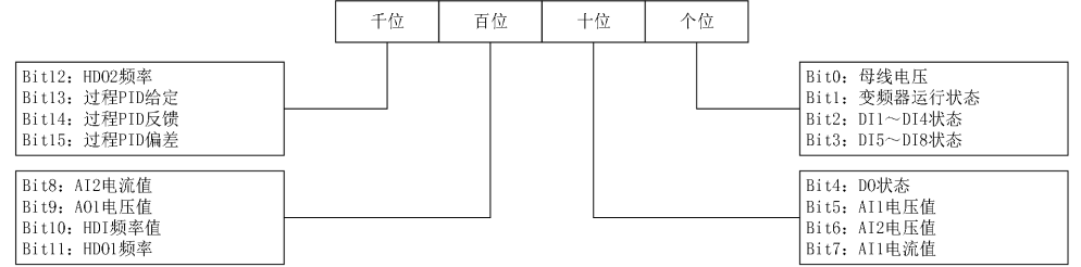
图7-49 LED运行显示参数选择2设定
