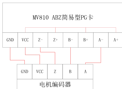
图 10-1 OC 接法
