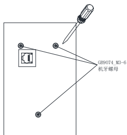
图c 简易安装
