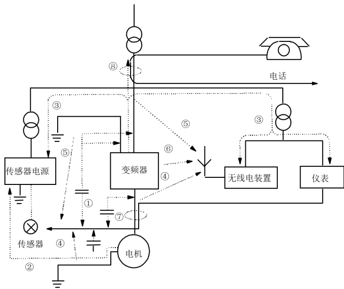
图 4-27 噪声传播路径示意图
