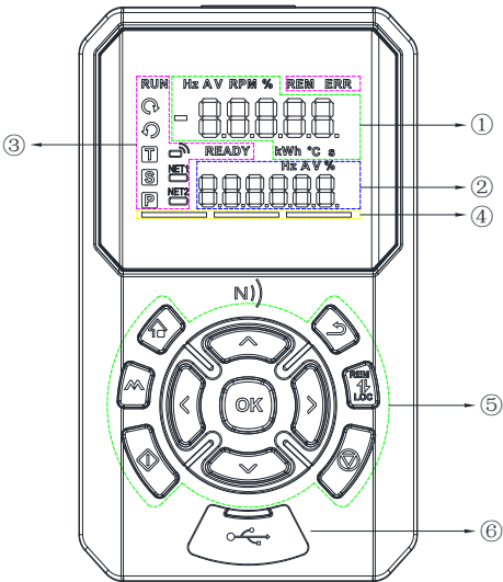
图 5-2 多功能键使用方法
