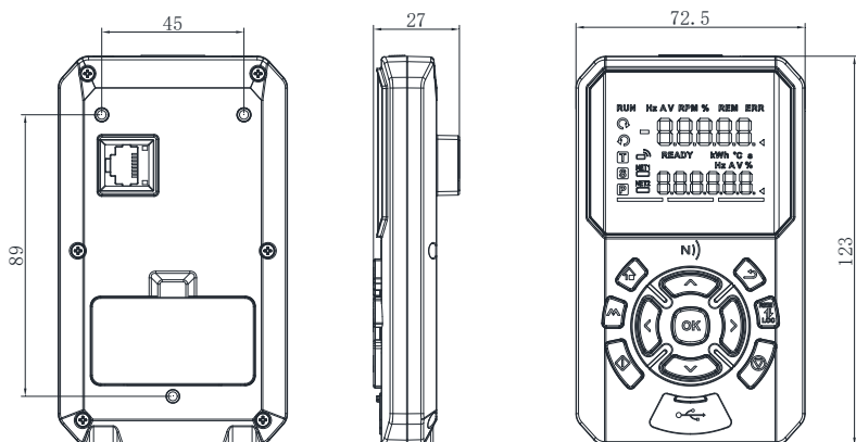
图2-49 大型远程LED键盘/操作面板（单位：mm）
