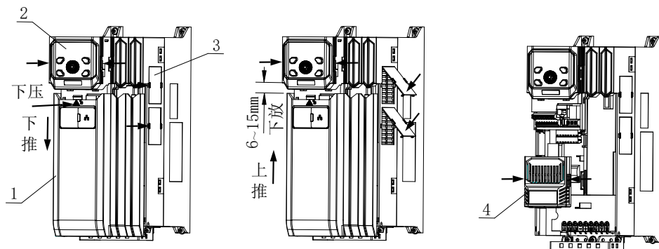
1: 盖板 2: 操作面板 3: 防尘盖 4: 扩展盒
