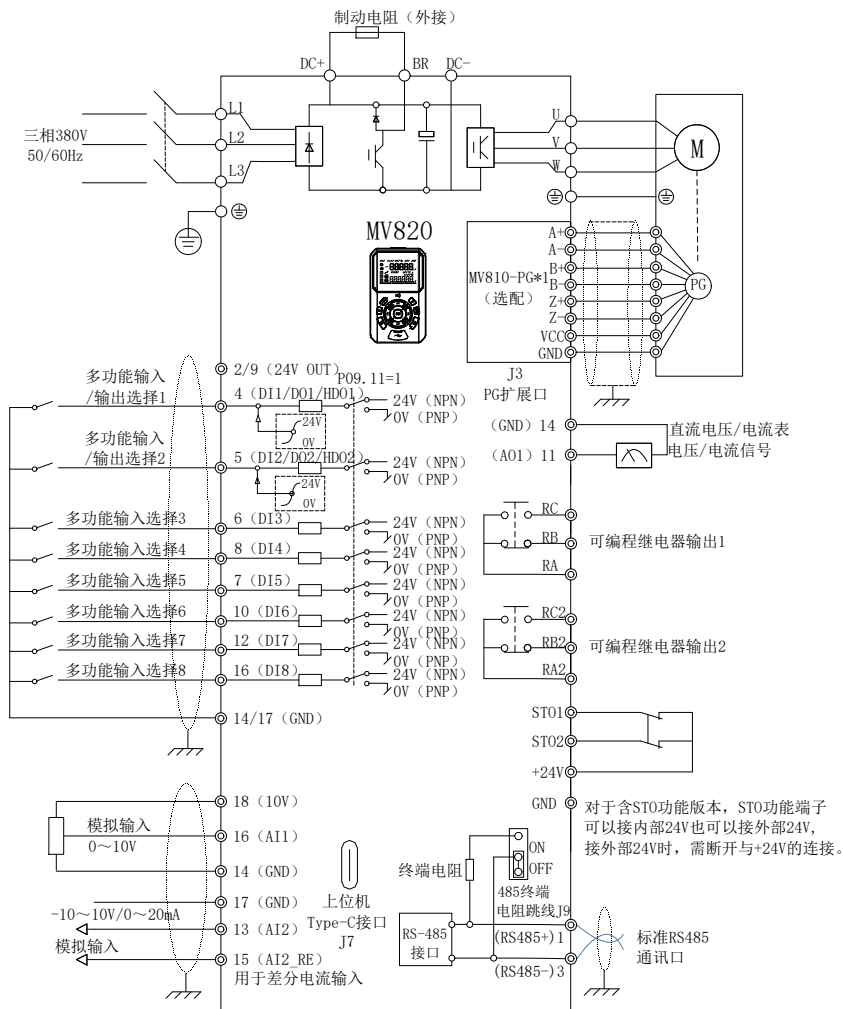
基本配线图 2
