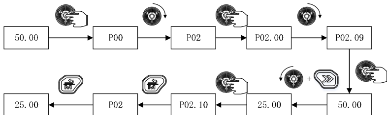
图 5-6 设置设定频率操作示例
