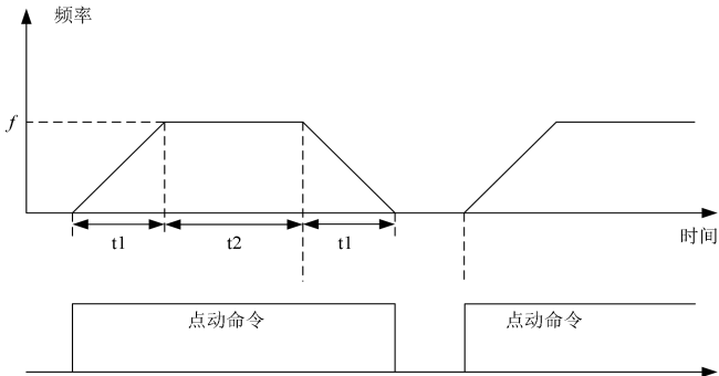
图7-30 点动运行参数说明
