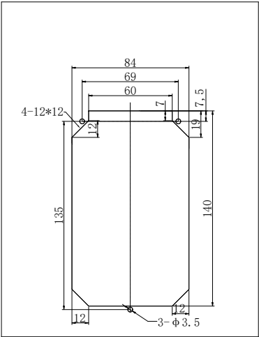
图2-46 大型操作面板固定座安装孔尺寸（单位：mm）
