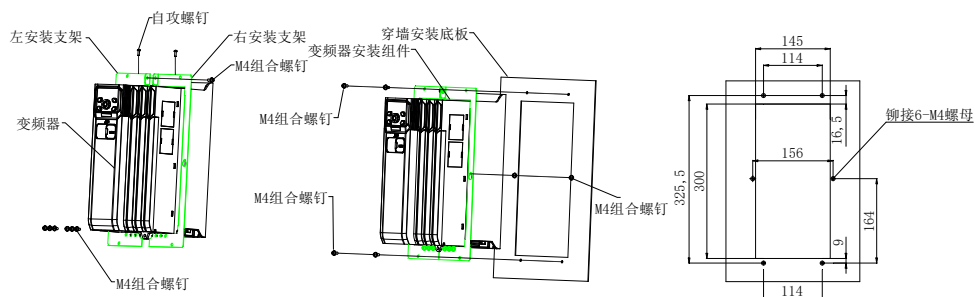
图2-35 MV810-EMBD (适用于11~15kW)
