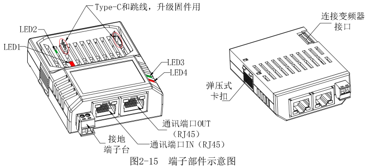
图2-15 端子部件示意图
