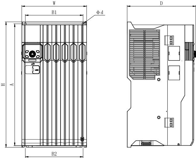
图 1-6 箱体 F
