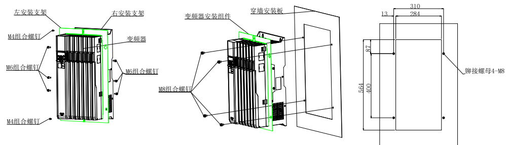
图2-38 MV810-EMBG (适用于45~75kW)
