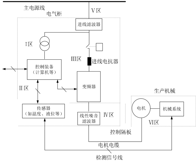
图 4-38 变频器 EMC 安装推荐区域划分示意图
