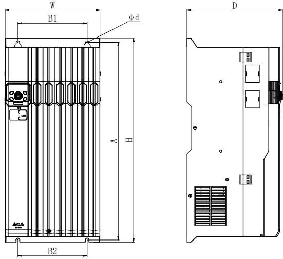
图 1-7 箱体 G
