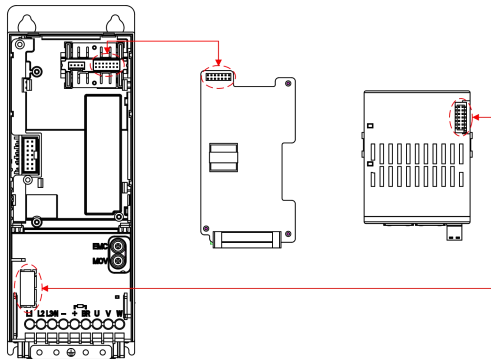
图2-2 电气接口示意图
