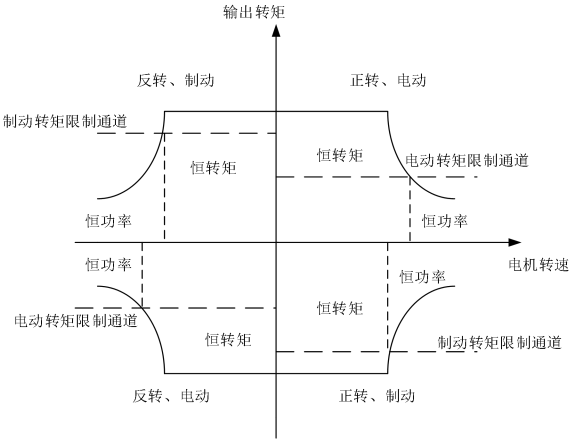
图7-13 转矩控制图
