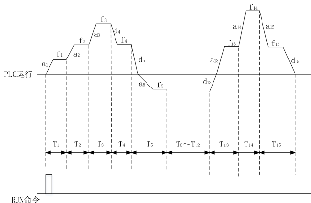
图7-36 PLC单循环后停机方式
