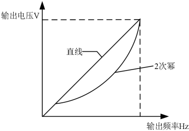
图 7-14 V/F 曲线
