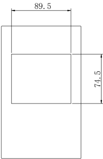
图2-44 操作面板固定座安装孔尺寸（单位：mm）
