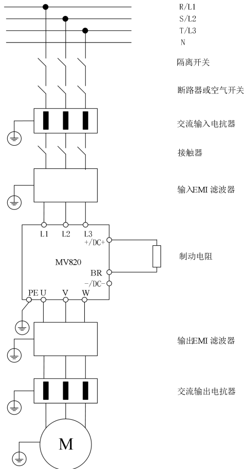
图 4-2 变频器与选配件的连接（以三相机型为例）
