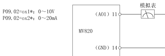
图 4-11 模拟输出端子配线
