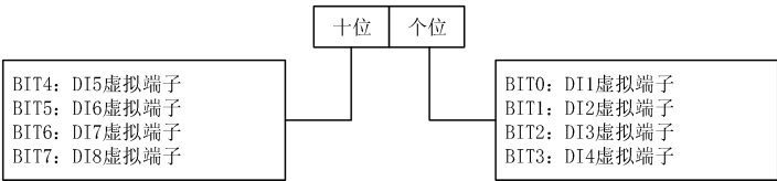
图7-23 虚拟输入端子设定
