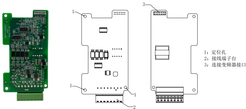
图2-18 外形及端子部件示意图
