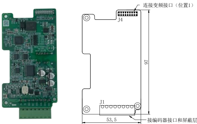
图2-25 外形及端子部件示意图
