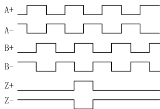
图2-20 ABZ信号波形图
