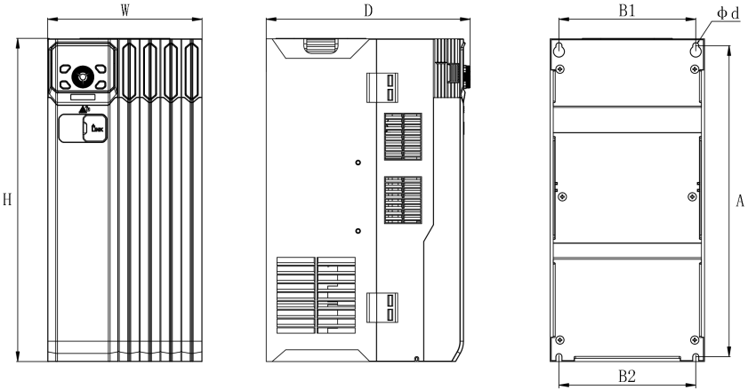
图 1-5 箱体 E
