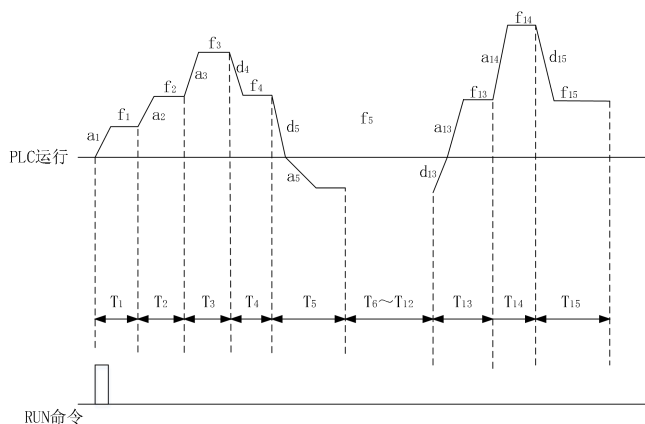
图7-37 PLC单循环后保持方式
