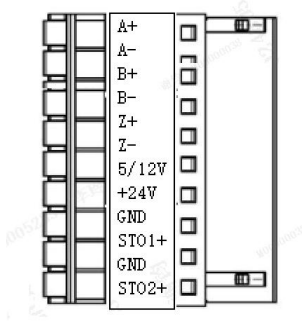
图附3-1 带 ST0 功能的PG卡端子
