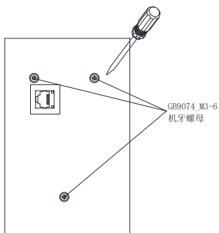
图c 简易安装
