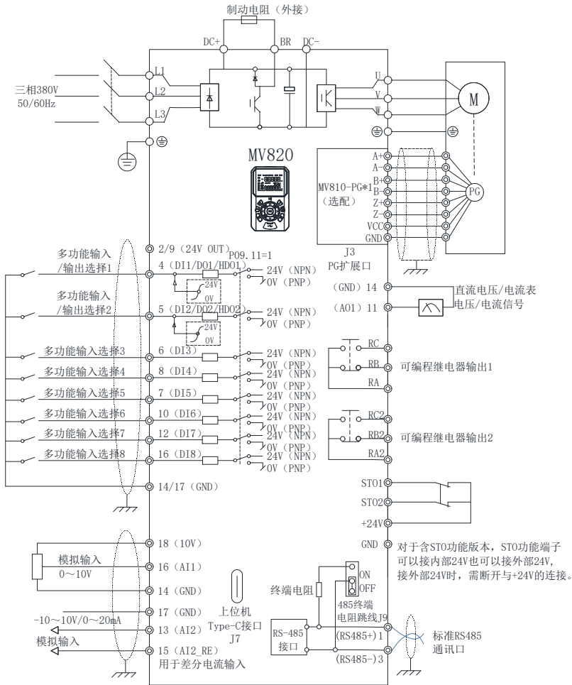
图 4-4 基本配线图 2
