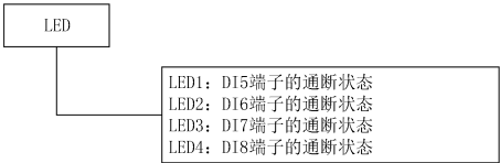
图7-4 开关量输入端子状态
