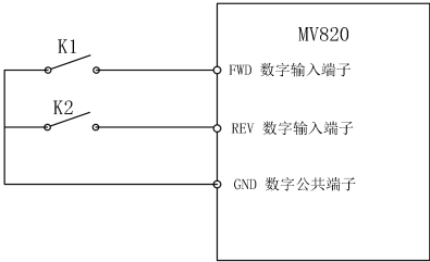
图7-19 两线式控制模式1
