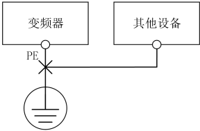
图 4-34 接地示意图 4
