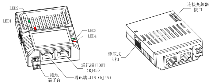
图2-32 产品外观
