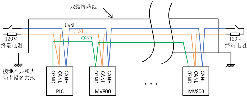
图2-14 ECAT总线连接示意图
