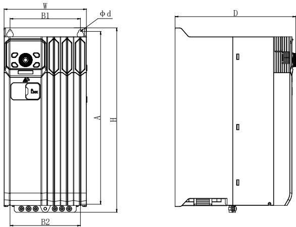
图 1-4 箱体 D
