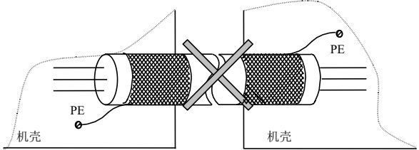
图 4-30 错误的屏蔽接地方法
