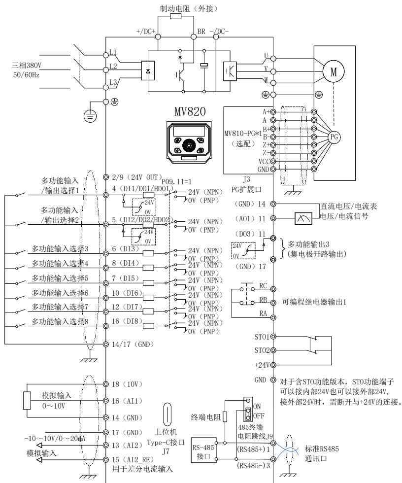
基本配线图 1
