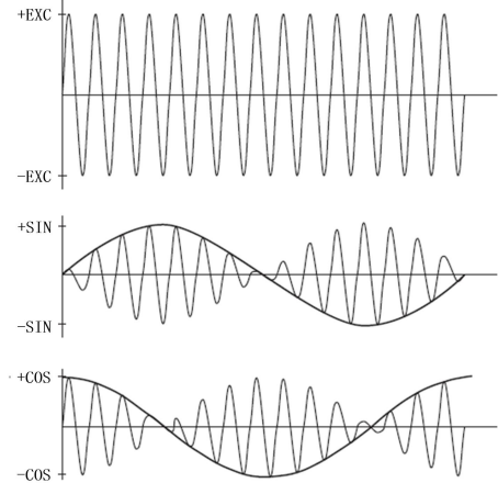
图2-27 旋变信号
