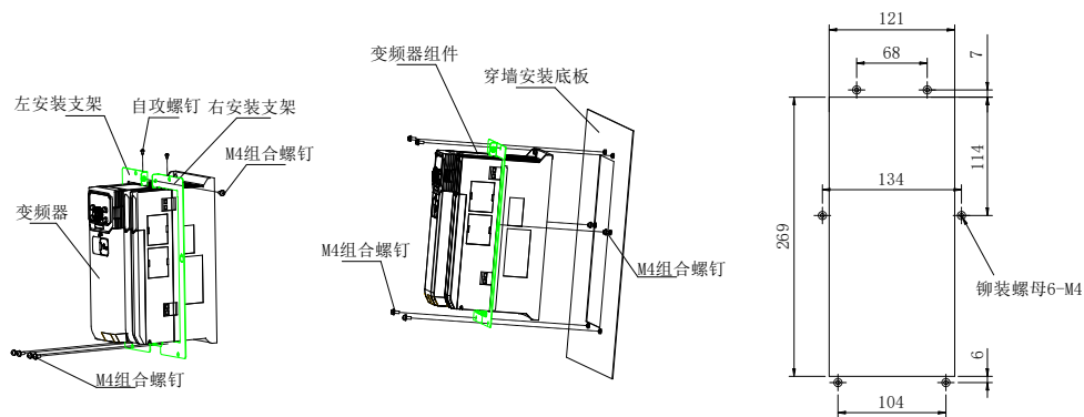
图2-34 MV810-EMBC (适用于5.5~7.5kW)
