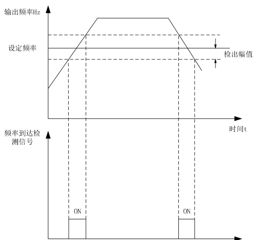
图7-32 频率到达 (FAR) 检出幅度
