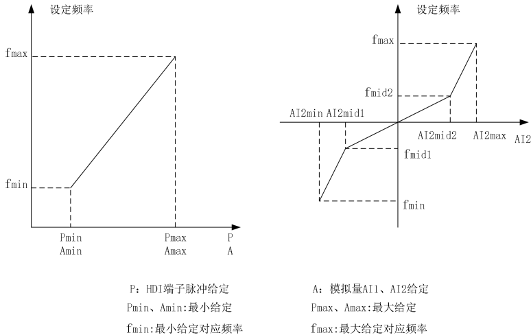
图7-25 模拟输入频率特性曲线
