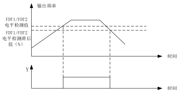
图7-33 频率水平检测示意图
