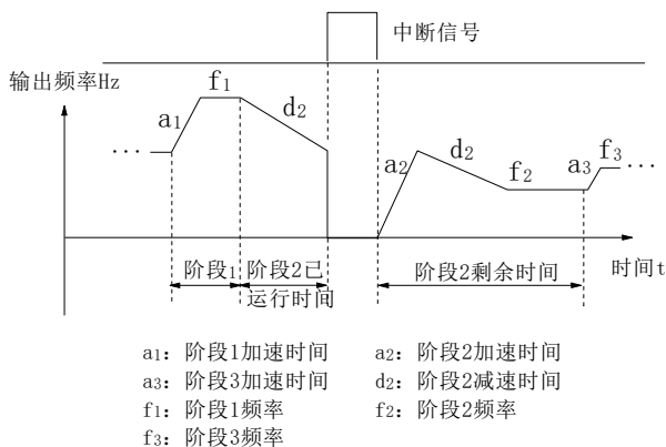
图7-39 PLC起动方式2
