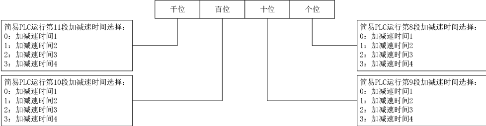
图7-42 简易PLC第8～11段加减速时间选择
