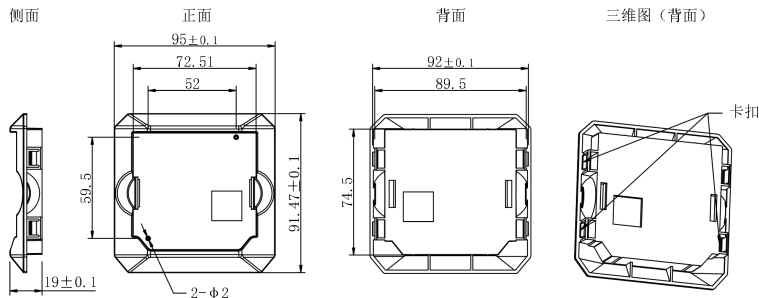
图2-43 键盘安装底座（单位：mm）
