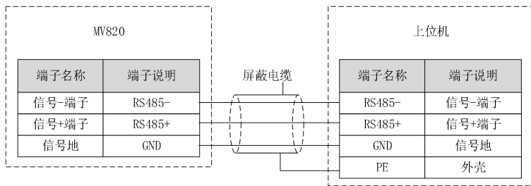
图 4-12 485-RS485 通讯配线
