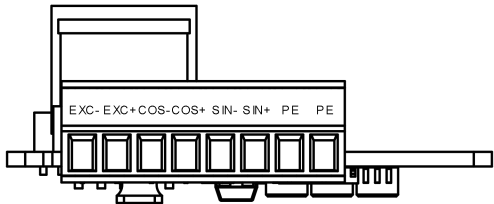
图2-26 端子丝印示意图
