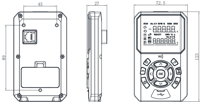
图 1-12 MV820-DP03 操作面板的外形和安装尺寸（单位：mm）
