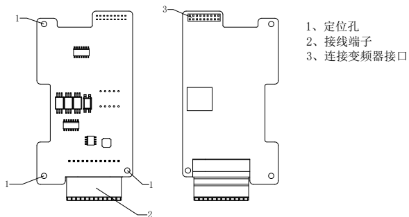
图2-21 外形及端子部件示意图(3.7kW及以下机型适配)
