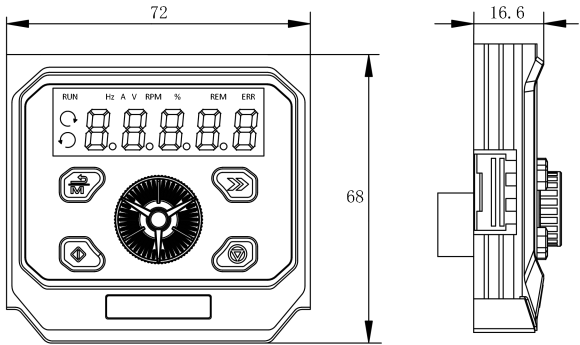
图 1-11 MV820-DP01 操作面板的外形和安装尺寸（单位：mm）
