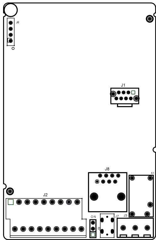
图 4-25 控制板示意图
