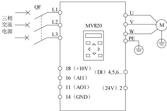
图 4-1 主回路简单配线图（三相机型）
