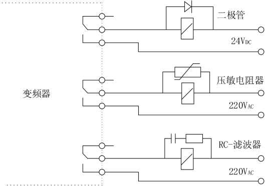
图 4-35 继电器、接触器及电磁制动器要求
