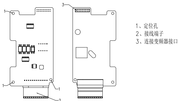
图2-22 外形及端子部件示意图 (5.5kW及以上机型适用)
