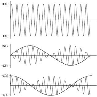
图2-31 旋变信号
