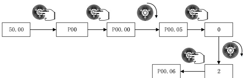
图 5-5 恢复出厂值设定操作示例
