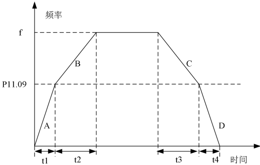
图7-29 加减速时间1、2切换示意图
